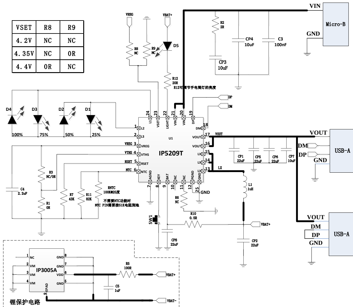
图 7 4LED 电量显示典型应用原理图
