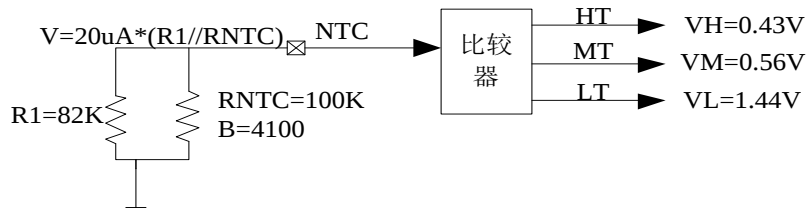
图 6 电池 NTC 比较
