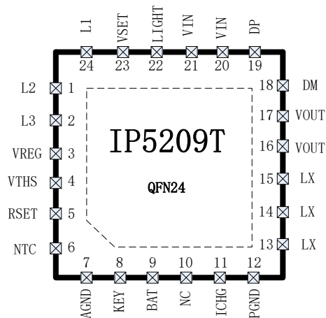
图 2 IP5209T 引脚图
