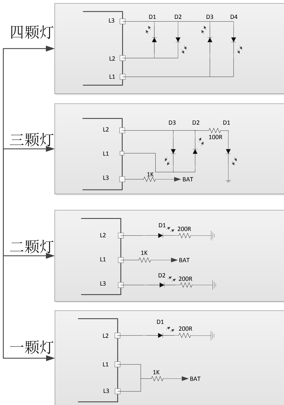
图 9 灯显模式
