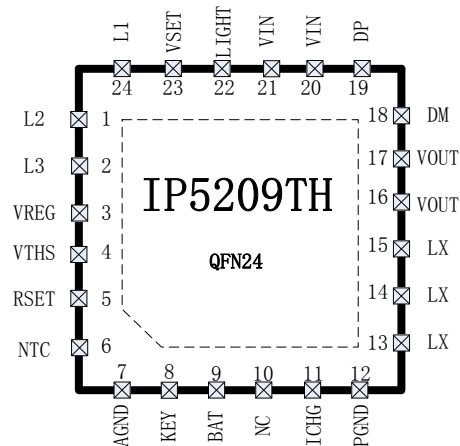
图 2 IP5209TH 引脚图
