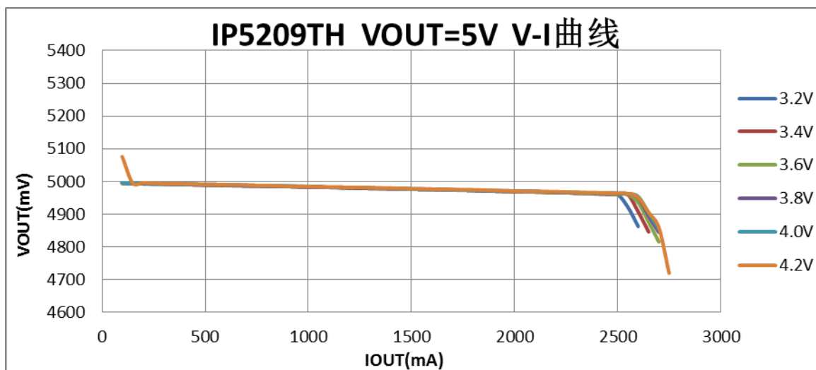
图 6 IP5209TH VOUT=5V V-I 曲线
