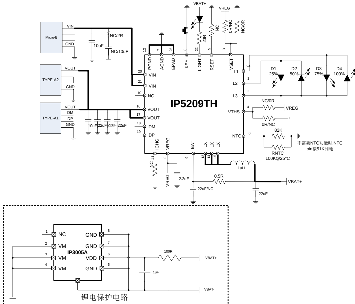
图 11 4LED 电量显示典型应用原理图
