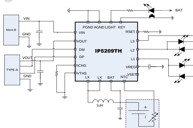
图 1 简化应用原理图(4 LED 指示电量)
