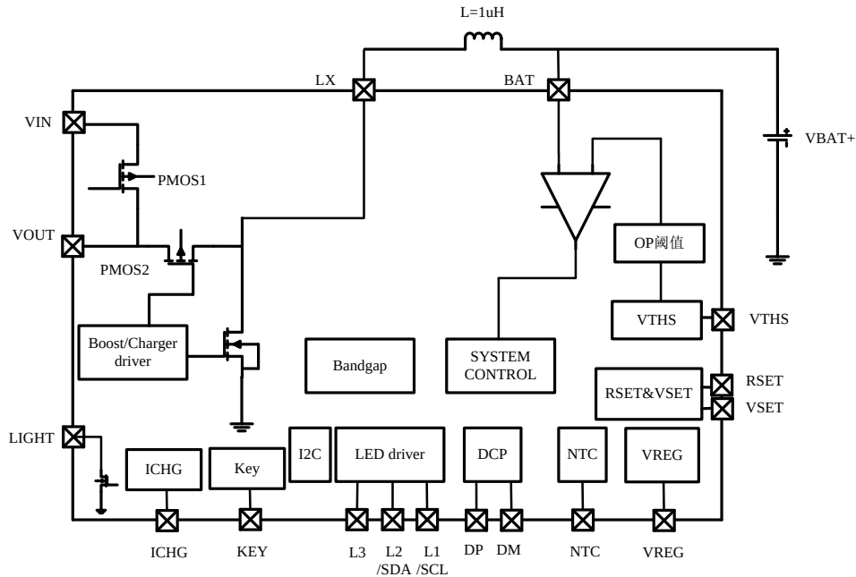
图 3 IP5209TH 系统框架
