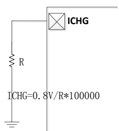
图 7 外挂电阻调节充电电流
