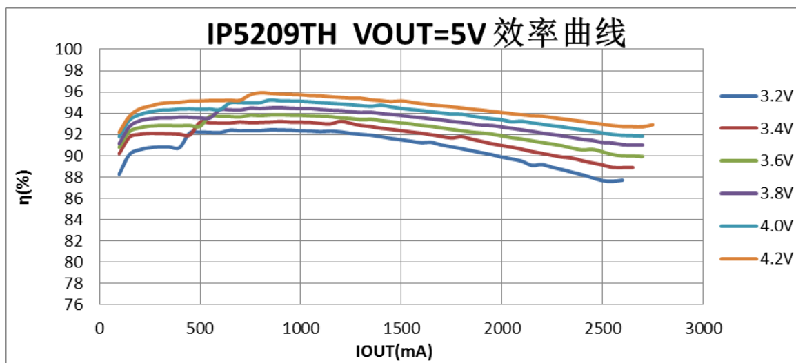
图 5 IP5209TH VOUT=5V 效率曲线
