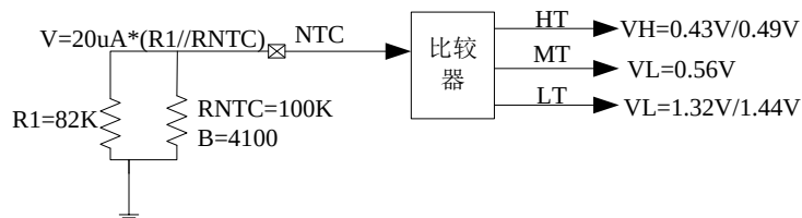
图 10 电池 NTC 比较
