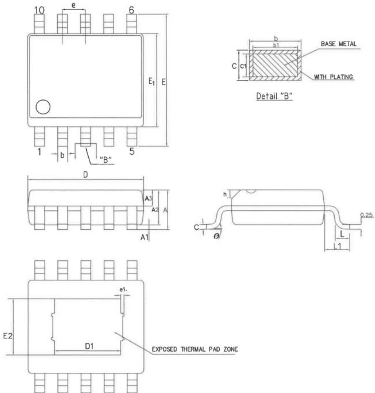
图 11 芯片封装
