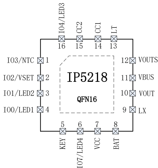
图 2 IP5218 引脚图
