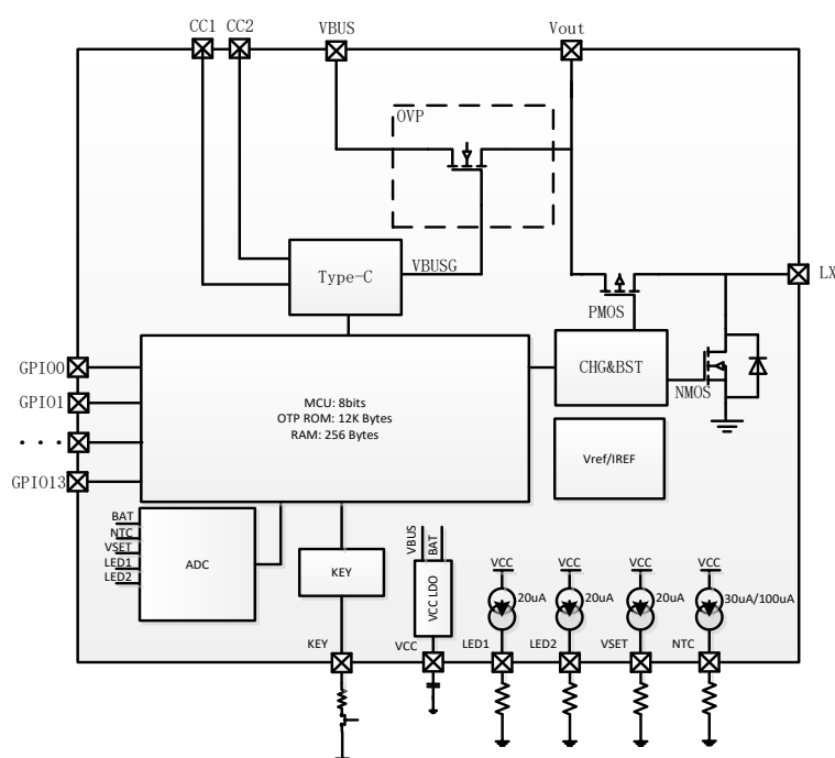
图 3 IP5218 内部系统框图
