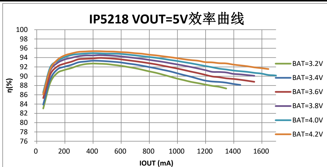
图4 IP5218 升压效率图
