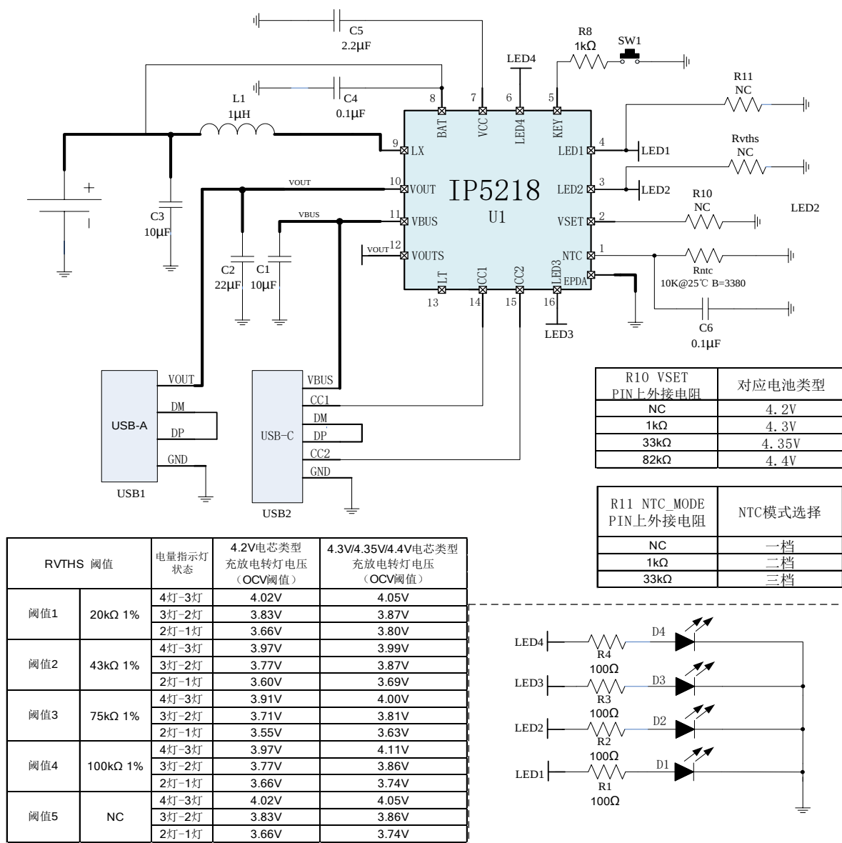
图 16 IP5218 典型应用原理图
