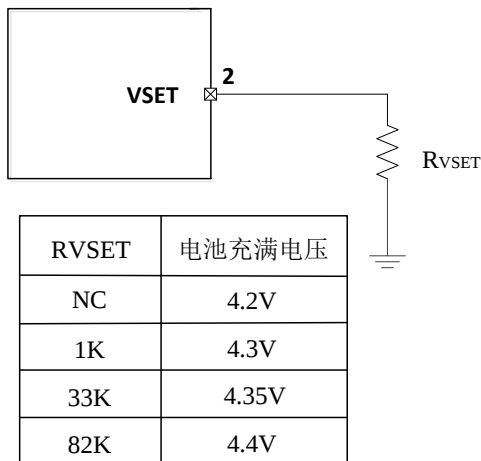
图 15 电芯电压 VSET 设置
