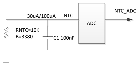
图 12 电池 NTC 比较
