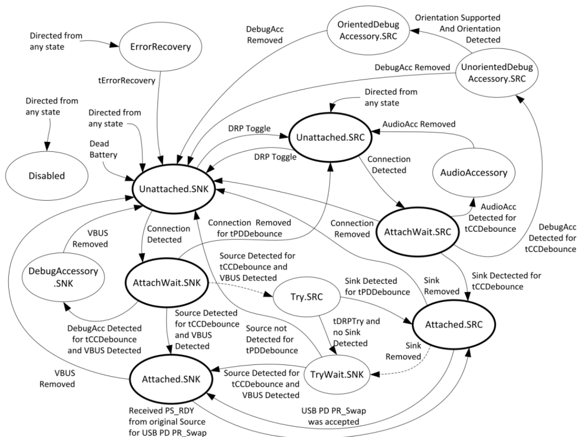
图 8 USB C 检测状态转换
