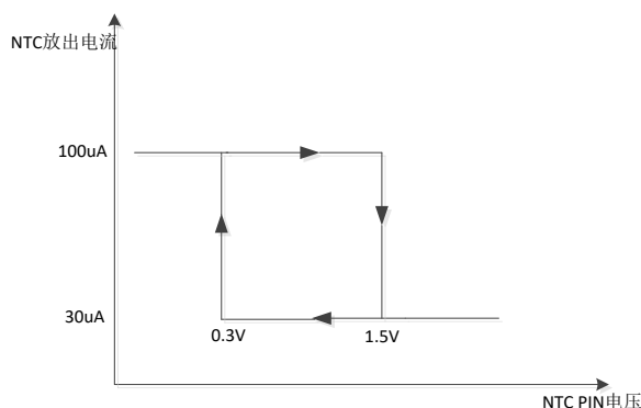
图 13 NTC 电压和放出电流关系
