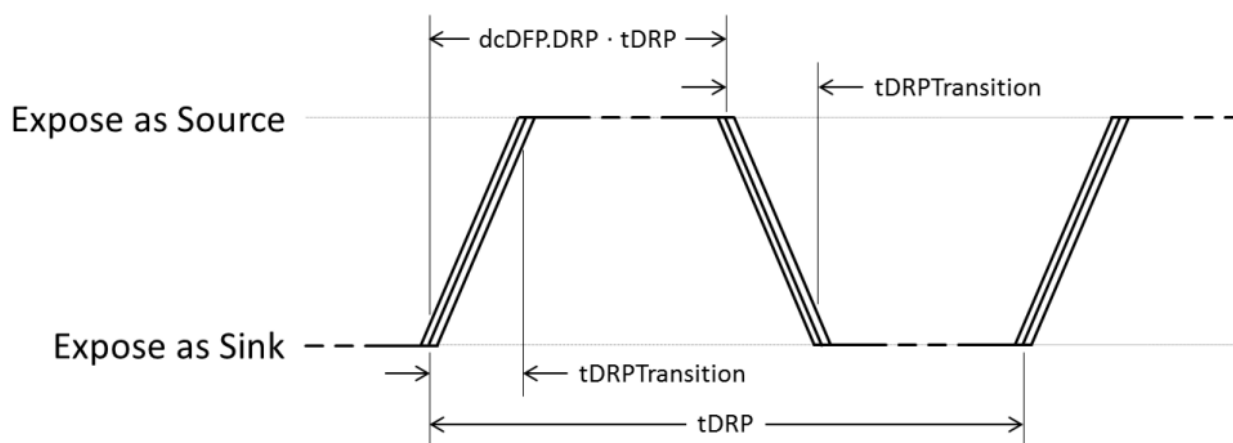
图 7 USB C 检测周期
