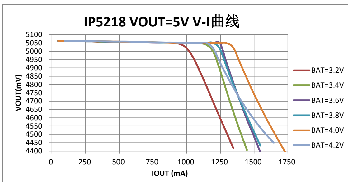
图5 IP5218 V/I 曲线图
