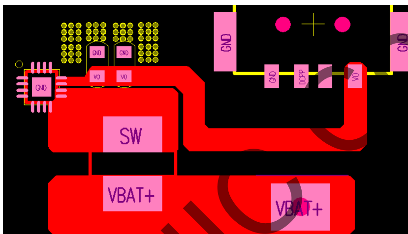
图 15 VOUT 电容
