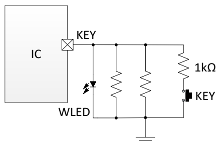
图 12 按键和照明
