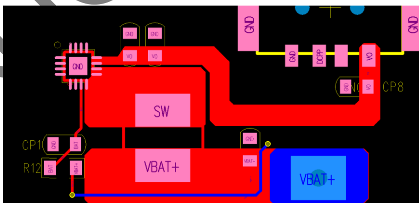
图 16 BAT 电容
