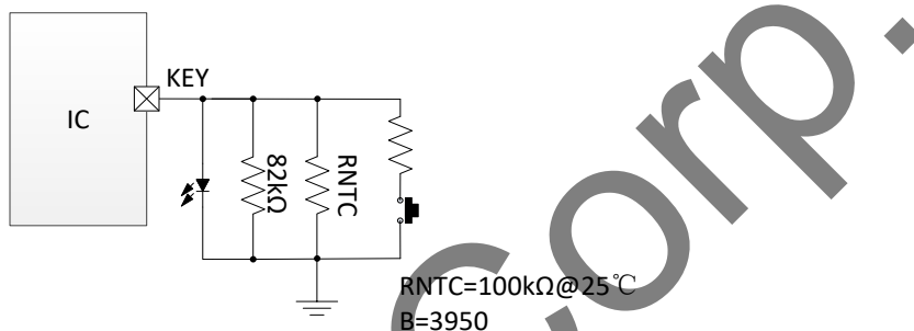
图 13 电池温度检测
