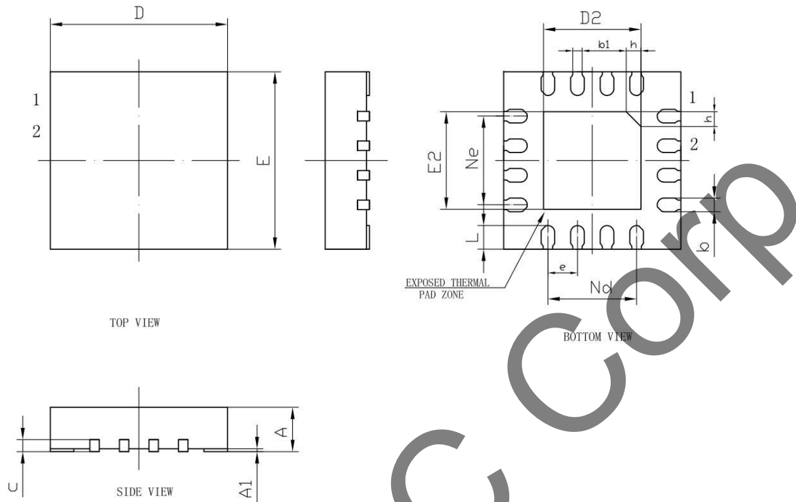
图 19 芯片封装
