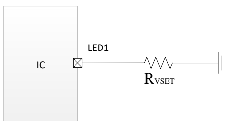
图 11 电池类型配置电路图
