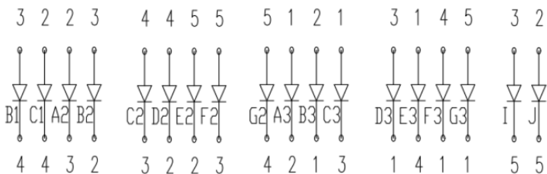
图 16 5 脚 188 型数码管电路图
