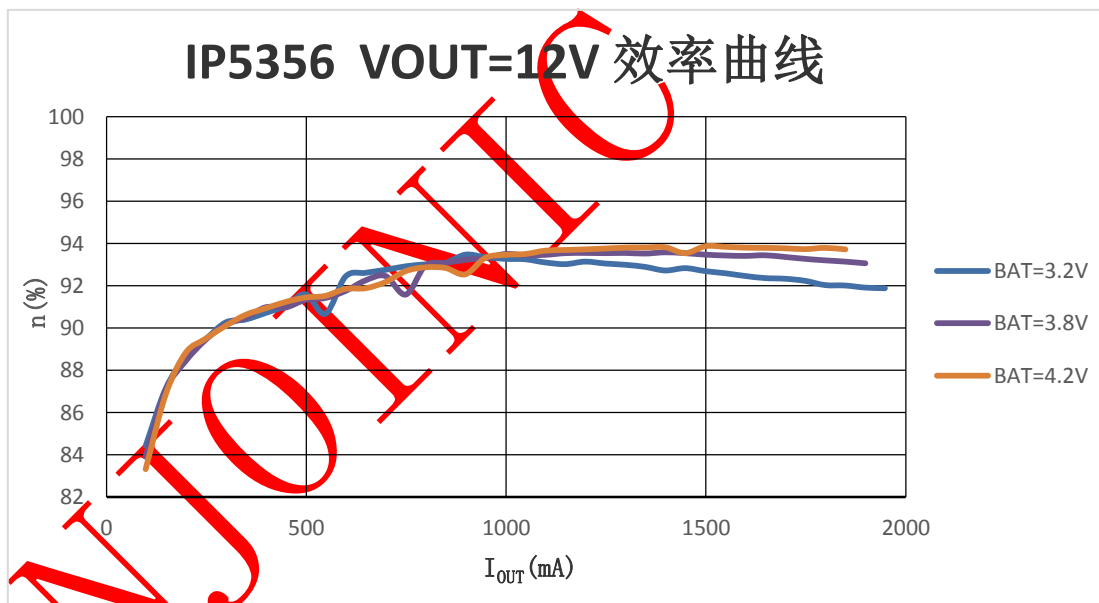
图 8 IP5356 VOUT=12V 效率曲线
