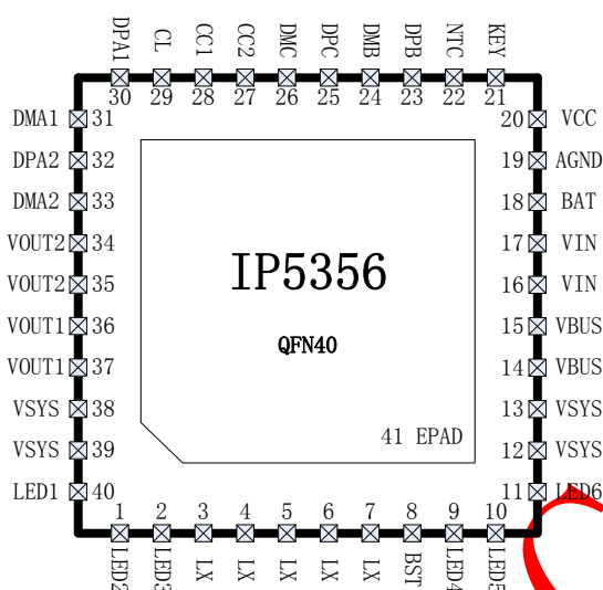
图 2 IP5356 引脚图
