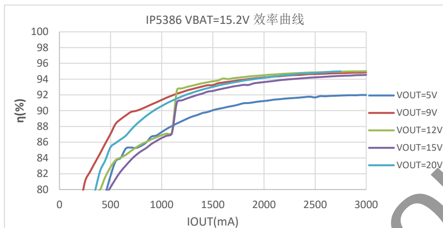
图 5 VBAT=15V 放电效率曲线图
