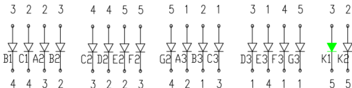
图 14 188 数码管 PIN 脚
