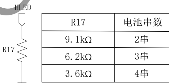
图 16 电池串数连接电路
