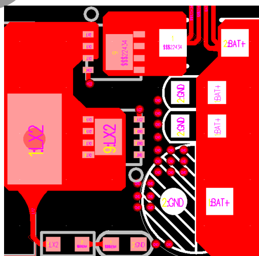
图 20 BAT 电容
