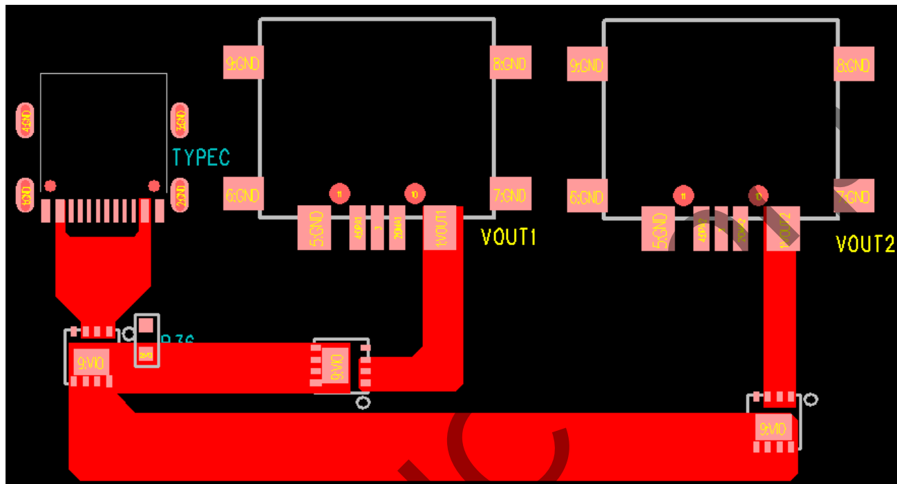
图 21 VIO 到各输出口走线
