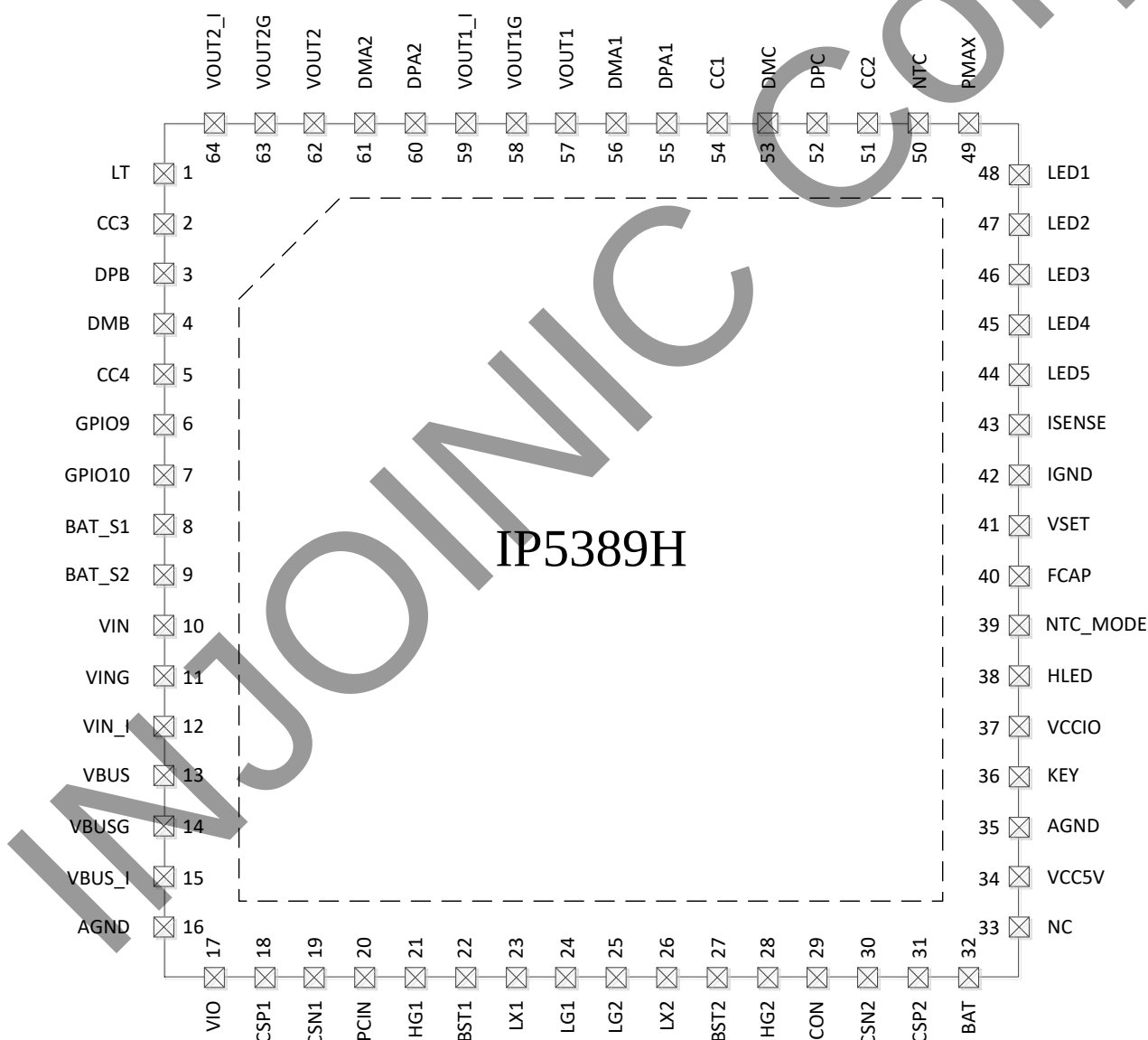
图 2 IP5389H 引脚图
