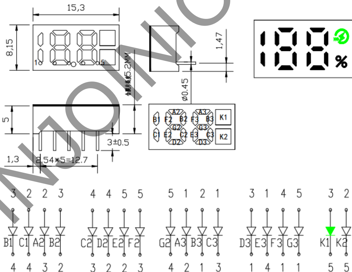
图 12 5pin 188 型数码管电路图
