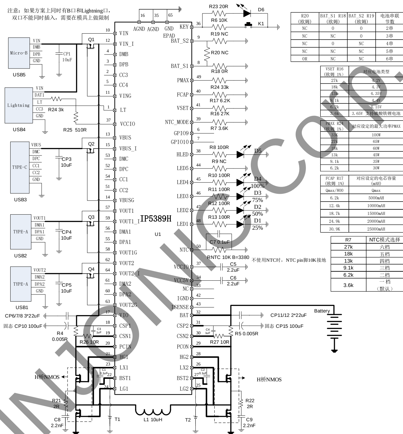
图 15 AABC 应用原理图
