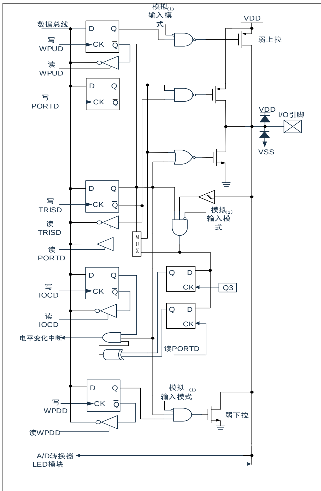
图 6-4: PORTD I/O 口结构图
