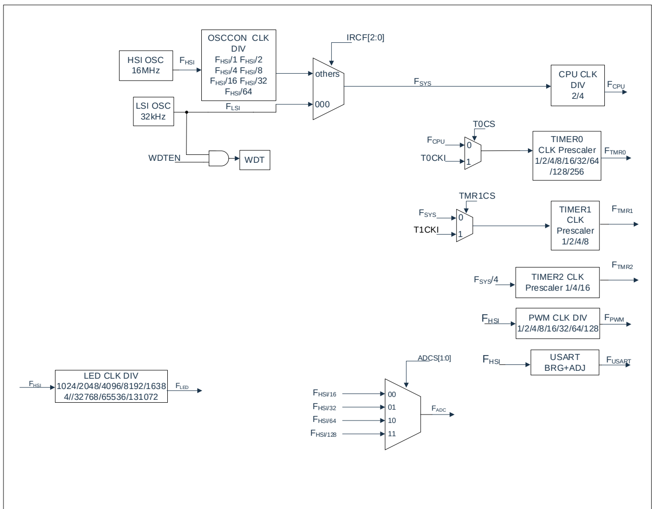
图 3-3: 时钟框图
