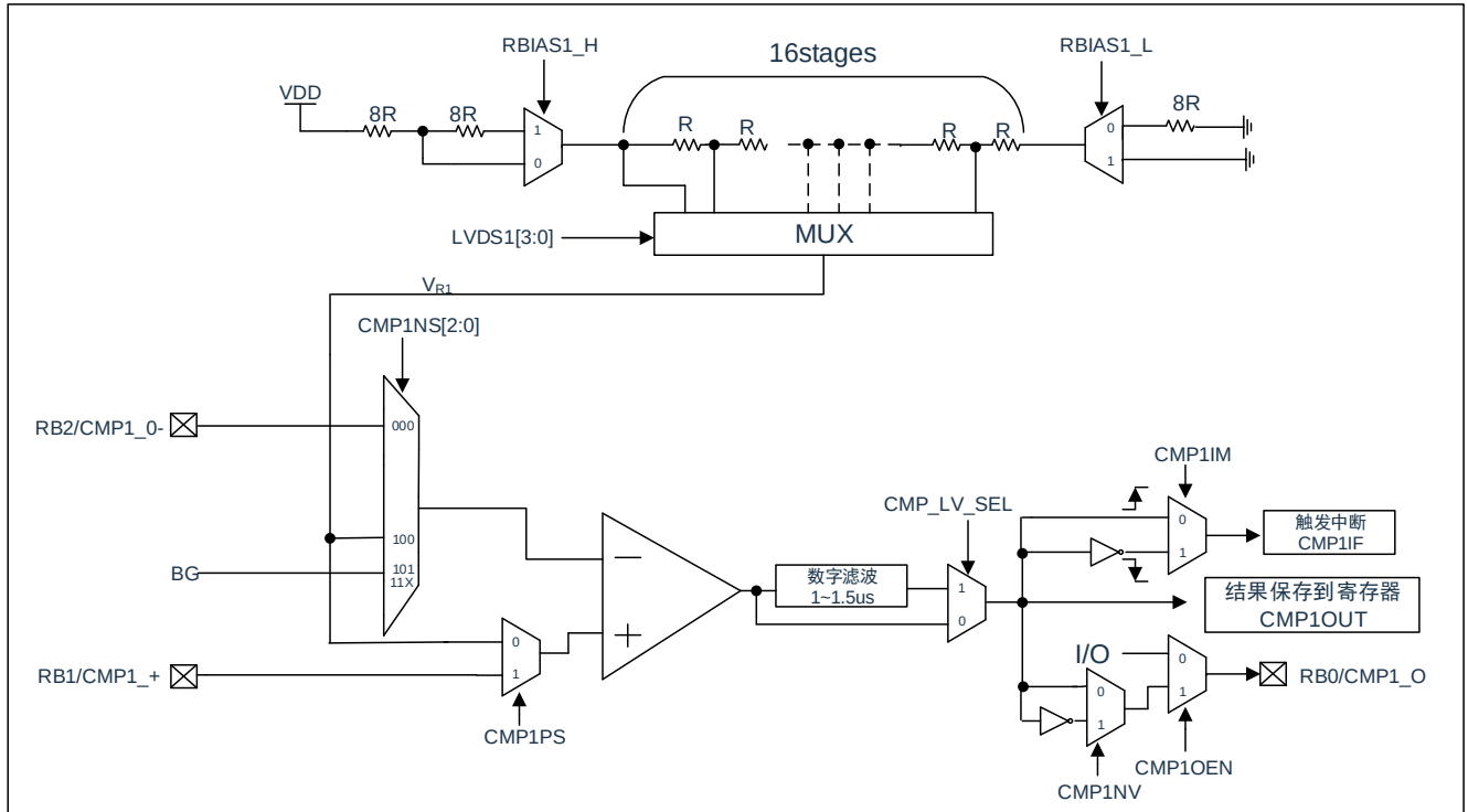
图 13-1: CMP1 的功能框图
