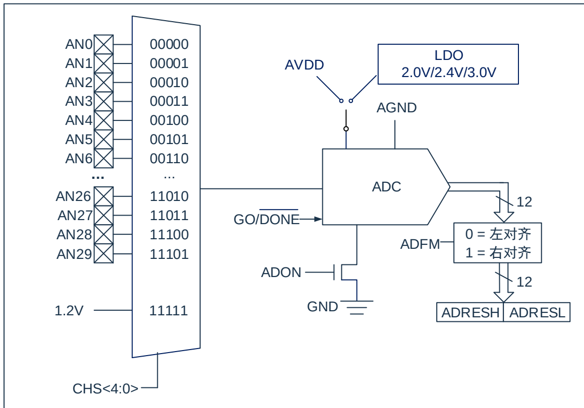
图 14-1: ADC 框图
