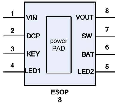
图 2 IP5406T 引脚图
