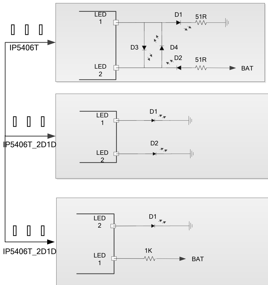
图 6 灯显模式
