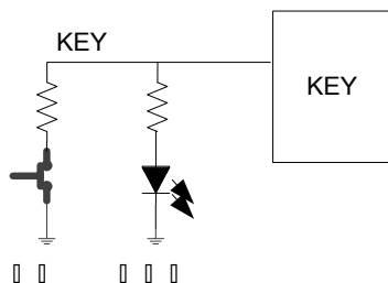
图 5 按键、照明灯示意图
