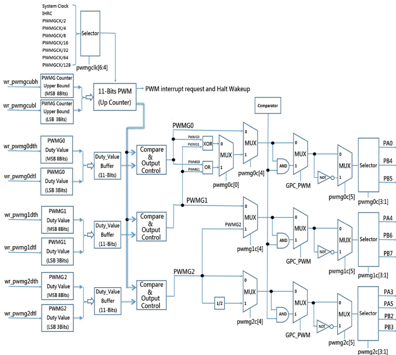
图.13：整组 SuLED 三路 11 位 PWM 生成器硬件方块图
