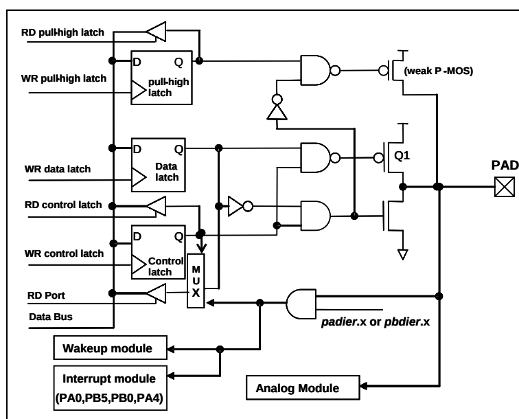
图.19：IO 引脚缓冲区硬件图
