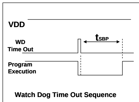
图.15：看门狗超时溢出时序图
