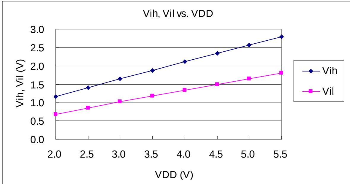
4.13. IO 引脚输入高/低阈值电压( V_{IH}/V_{IL} )曲线图
