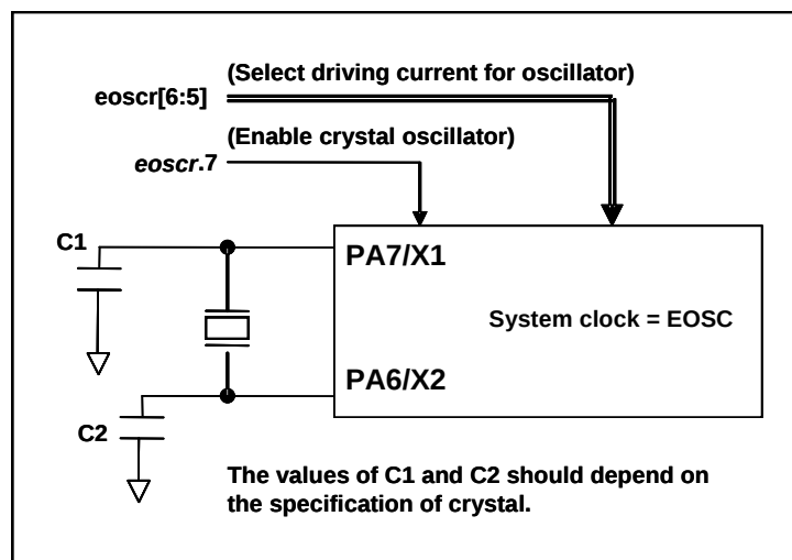
图.2： 晶体振荡器的硬件连接图
