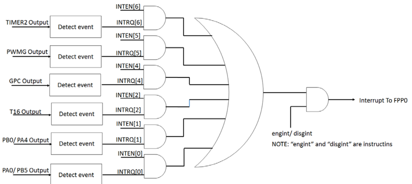
图.16： 中断控制器硬件框图
