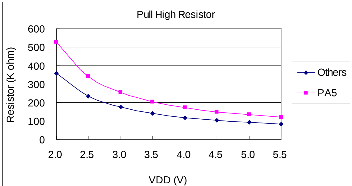
4.14. IO 引脚上拉阻抗曲线图
