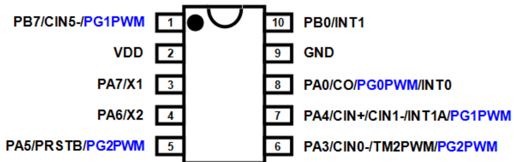
PMS152-M10 (MSOP10-118mil)
