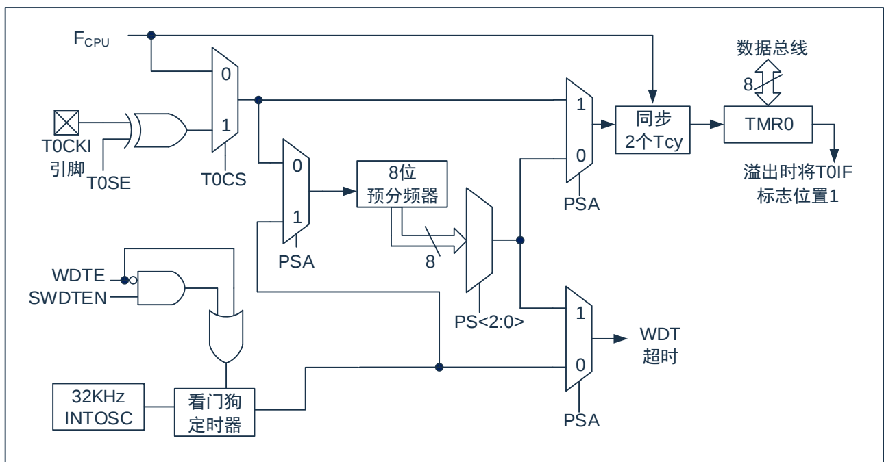
图 8-1: TIMER0/WDT 结构图
