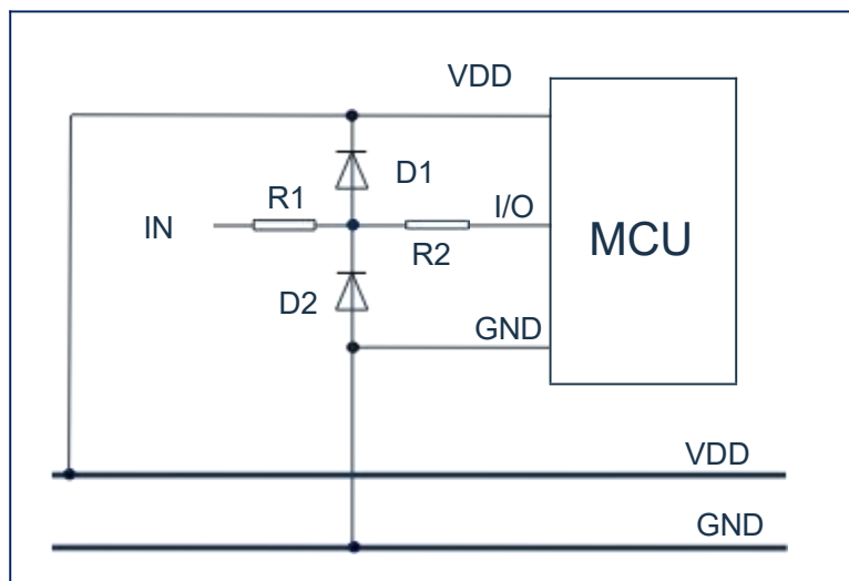
图 6-2: I/O 口注意事项连接图
