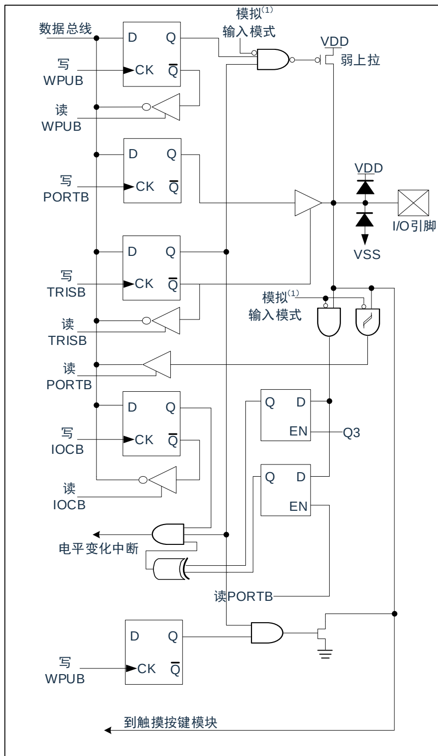
图 6-1: I/O 口结构图
