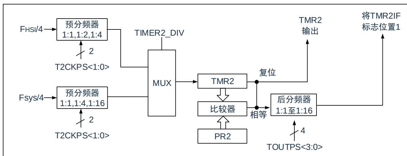
图 9-1: TIMER2 框图
