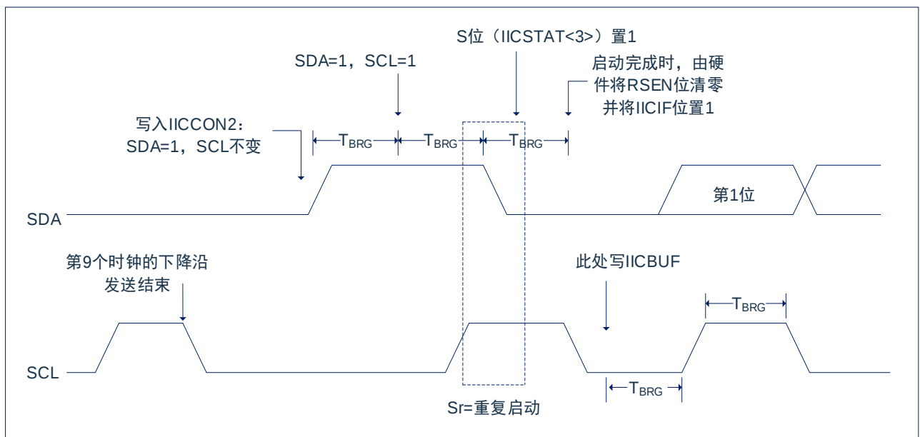
图20-8：重复启动条件时序波形
