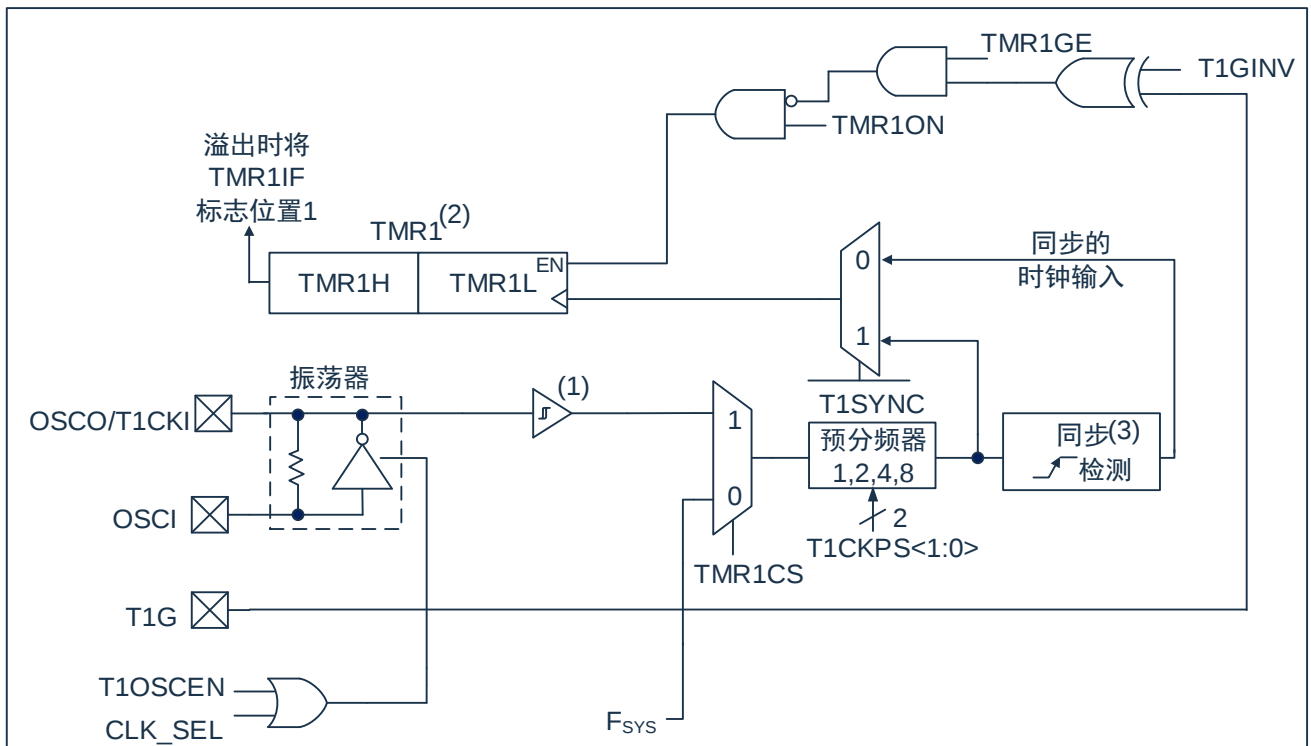
图9-1: TIMER1结构图
