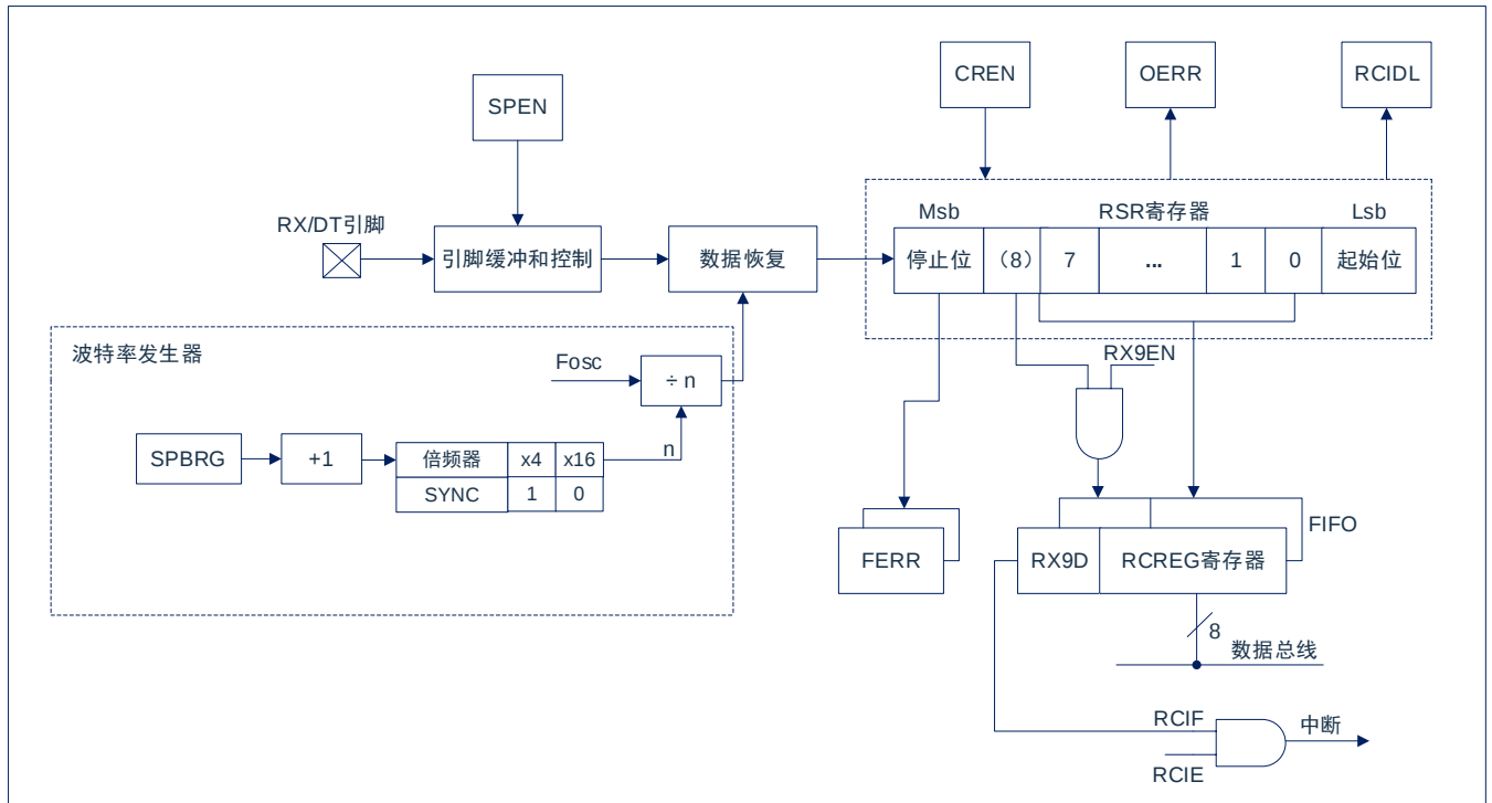
图18-2: USART接收框图
