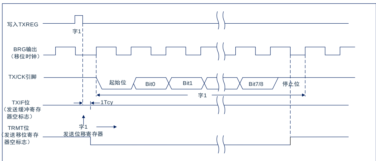
图 18-3: 异步发送
