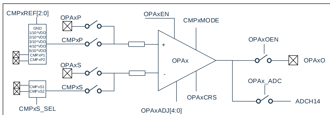
图 16-1: OPAx 框图
