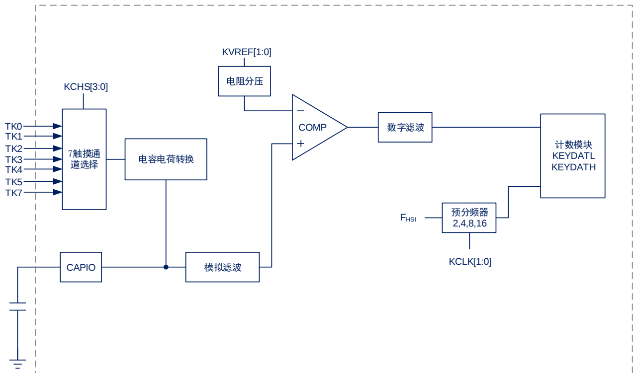
图21-1：内部电路框图
