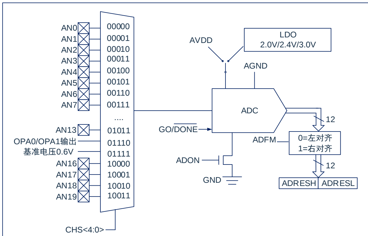
图 11-1：ADC 框图
