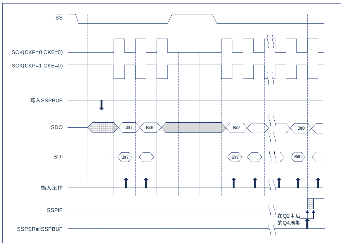
图 17-3：从动同步波形
