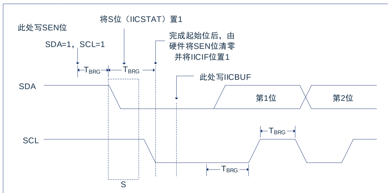
图18-7: 第一个启动位时序
