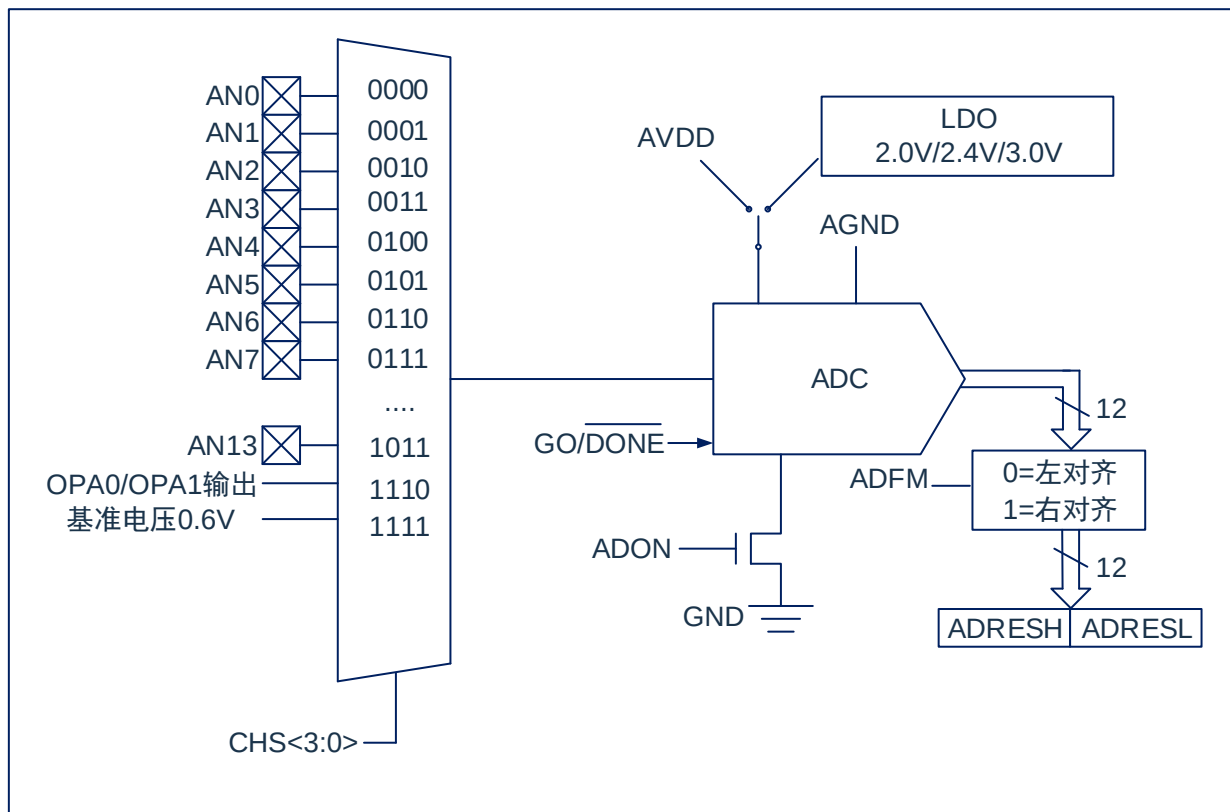
图 10-1: ADC 框图
