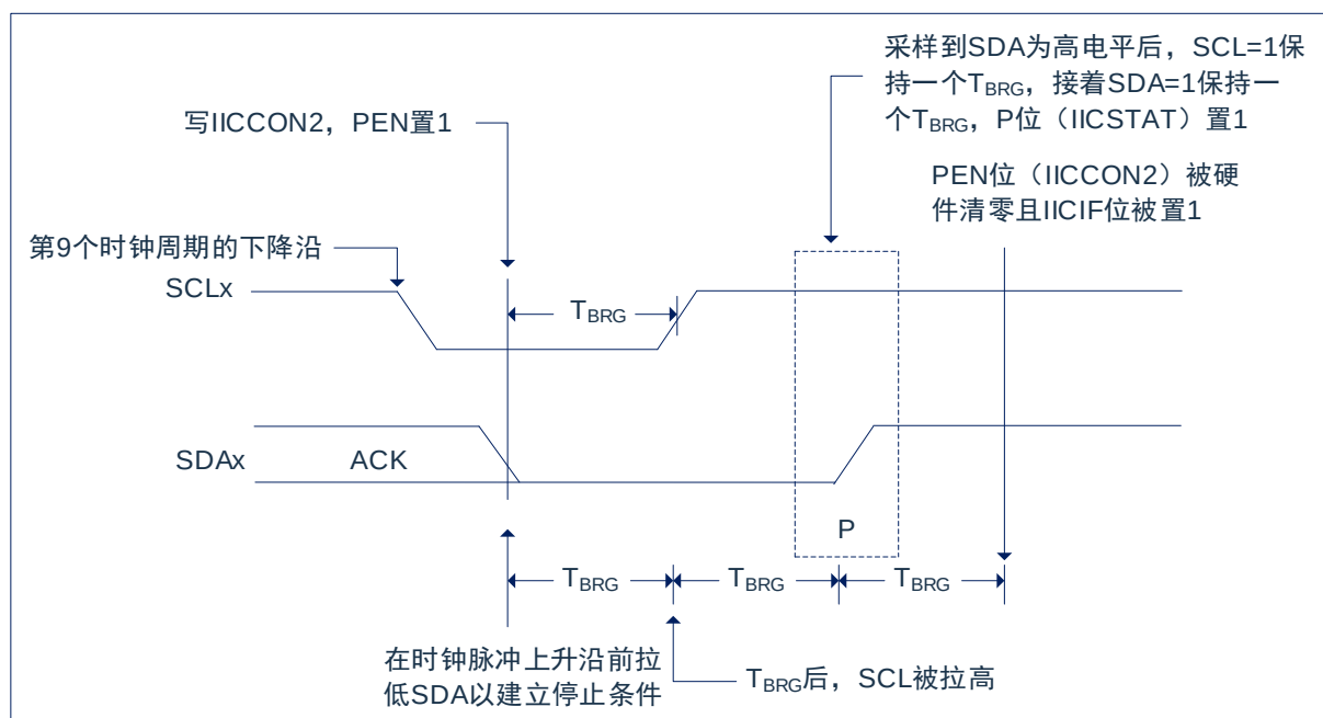
图 18-10：停止条件接收或发送模式
