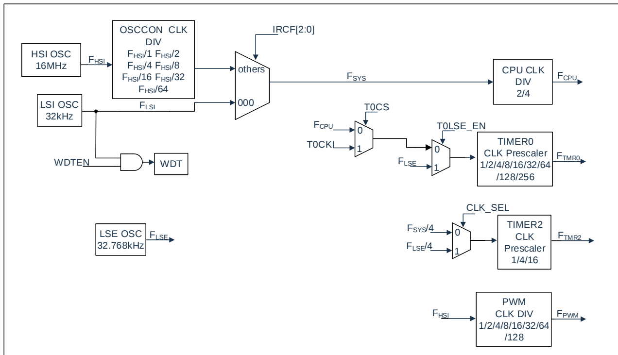
图 3-3: 时钟框图
