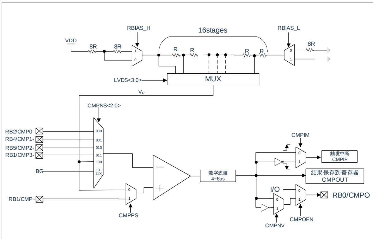
图 11-1：比较器的功能框图
