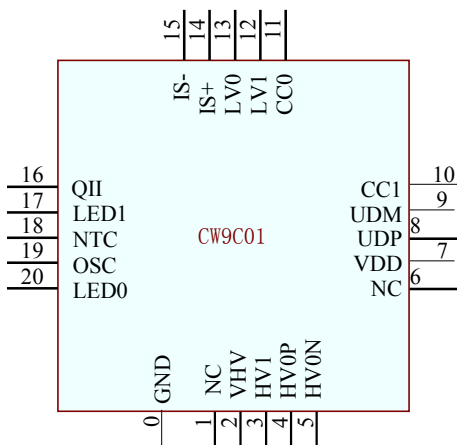
CW9C01 (QFN20_3*3) 封装引脚排列
