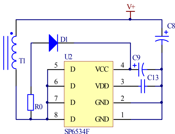
图 4 VCC 正反激供电电路
