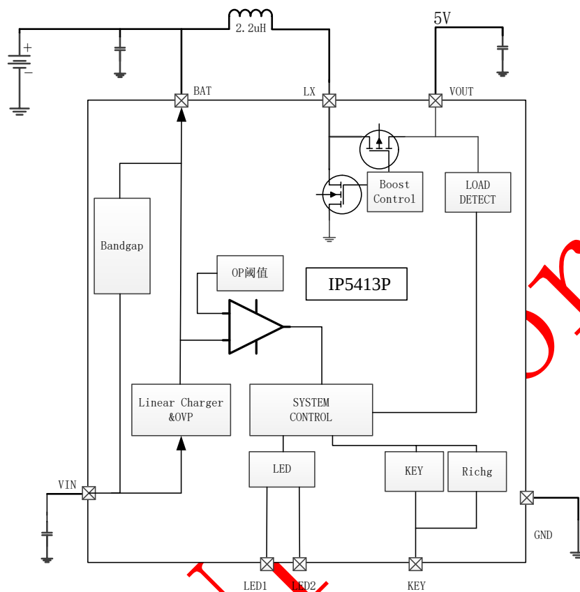
图3 IP5413P 内部系统框图
