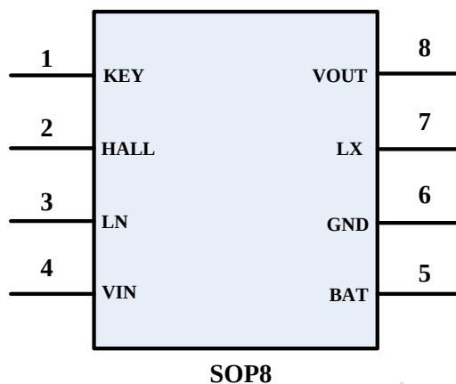
图 2 IP5416 引脚图
