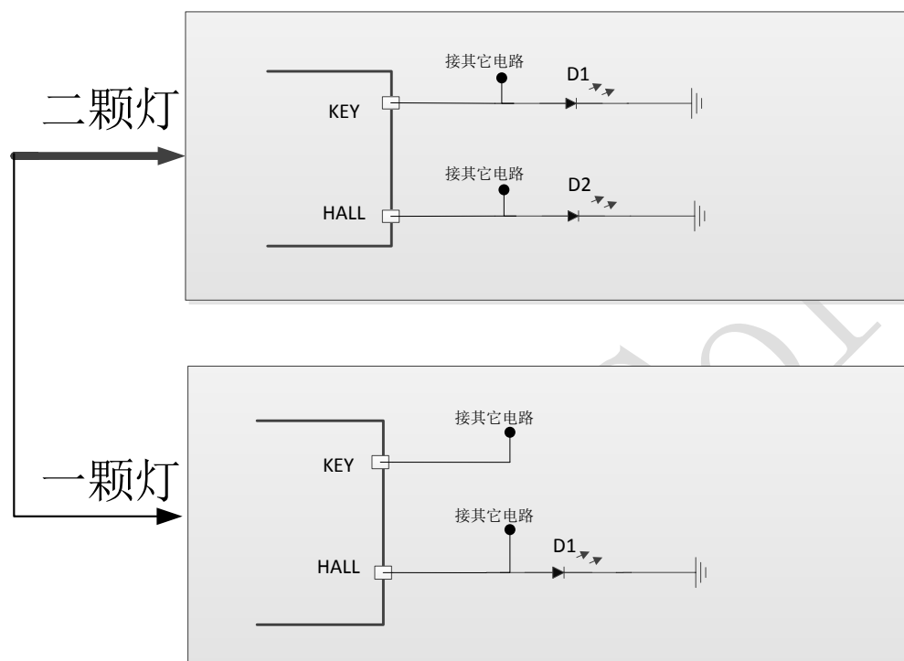
图 7 LED 显示配置电路图
