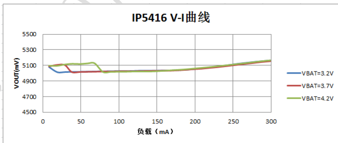
图 5 IP5416 V-I 曲线图
