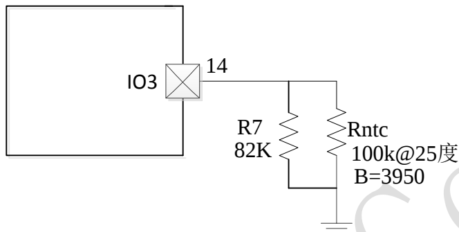
图9 NTC 电路图
