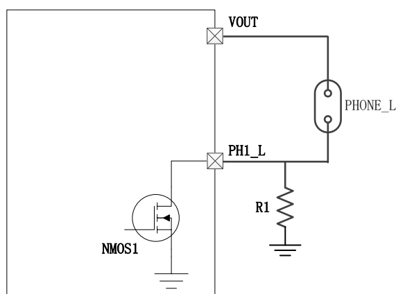
图 9 IP6838 耳机待机状态的电阻调节原理图
