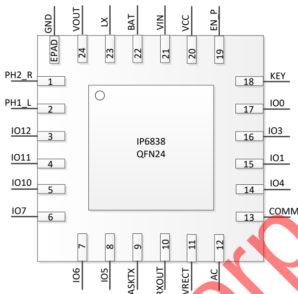
图 2 IP6838 引脚图
