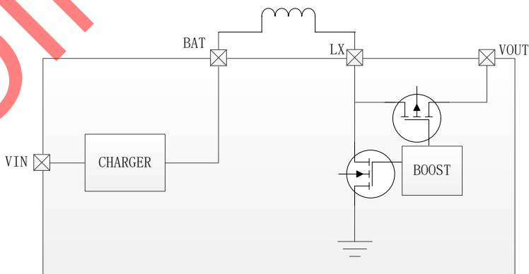
图 6 IP6838 路径管理示意图
