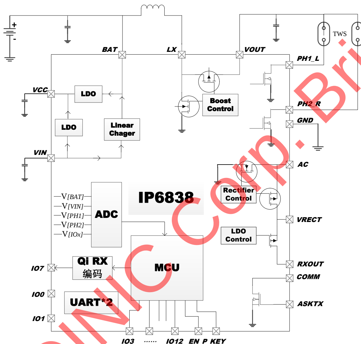
图 3 IP6838 内部系统框图
