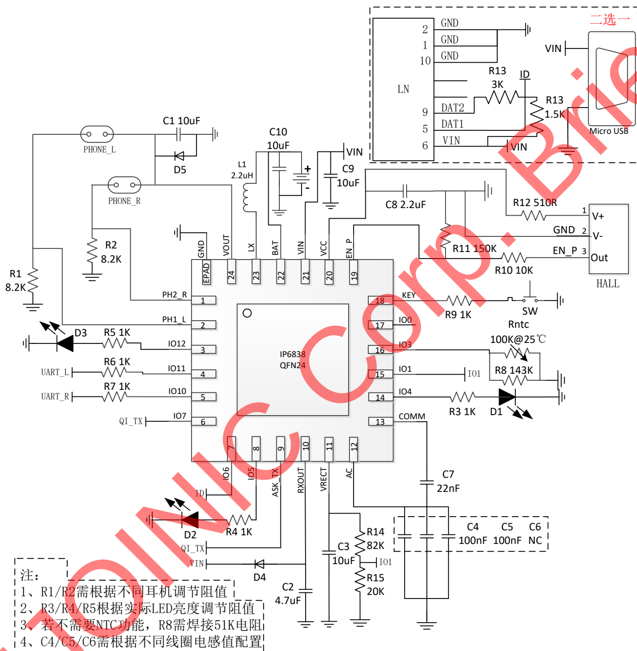
图 10 IP6838 TWS 负端通信应用的典型原理图
