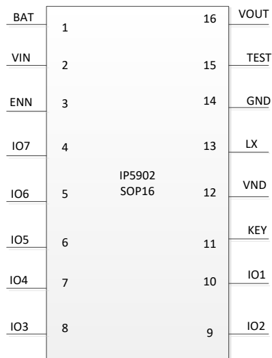
图 2 IP5902 引脚图
