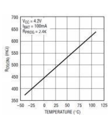
功率 MOS 开态电阻 vs 温度
