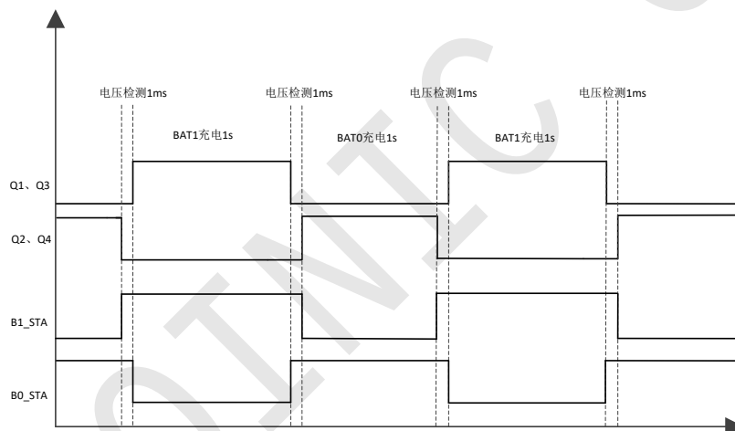
图 7 STA2 状态( -V_{TH}<V_{BAT1}-V_{BAT0}<V_{TH} )充电检测示意图
