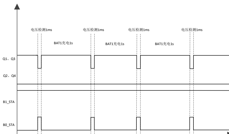
图 8 STA3( V_{BAT0}-V_{BAT1}>V_{TH} )状态充电检测示意图
