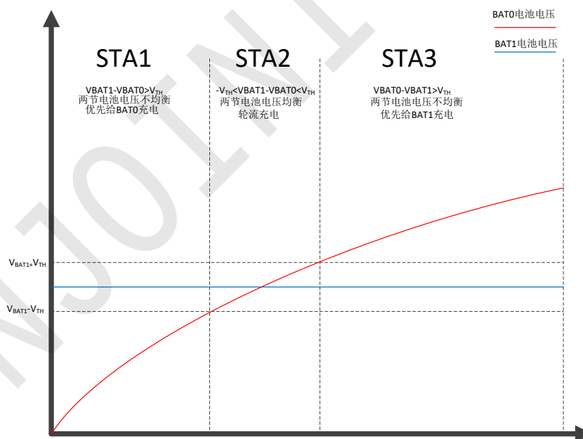
图 5 IP2305 电池切换策略示意图
