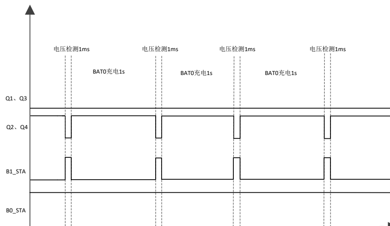
图 6 STA1 状态( V_{BAT1}-V_{BAT0}>V_{TH} )充电检测示意图
