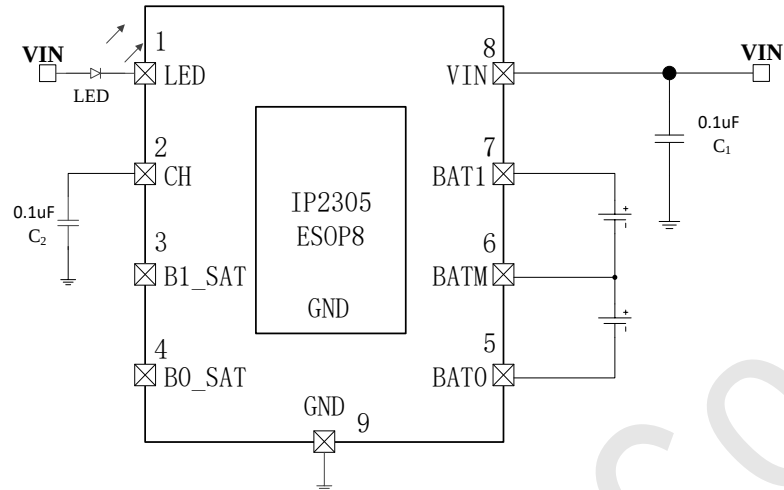
图 11 典型应用原理图
