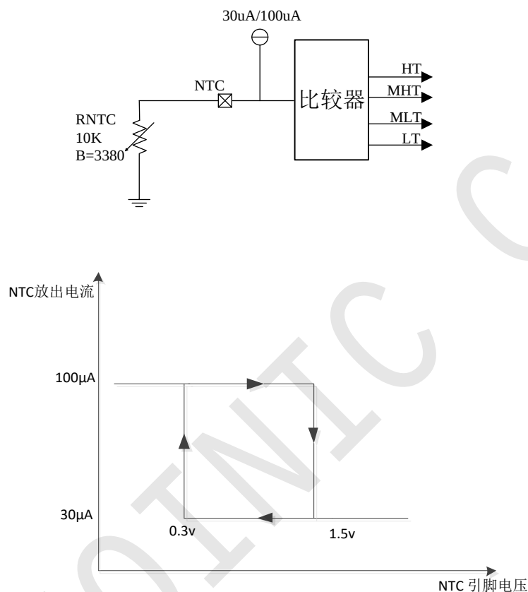
图 7 NTC 框图
