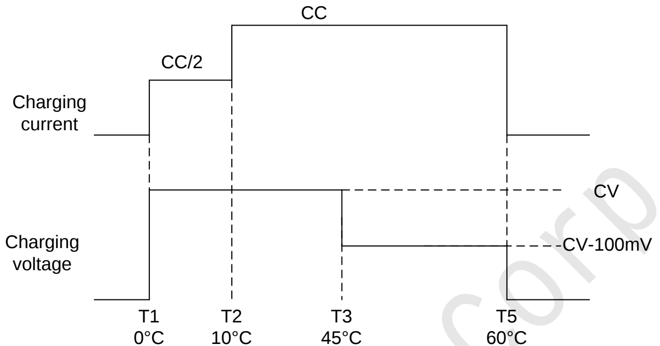
图 8 5 段式电池温度充电保护（兼容 JEITA 标准）示意图
