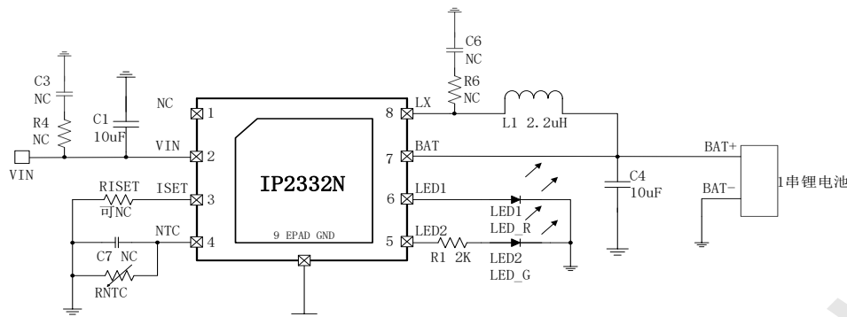
图 9 典型应用原理图
