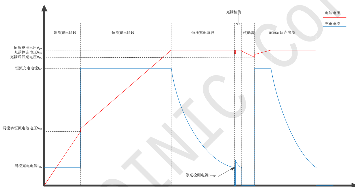
图 6 IP2332N 充电过程示意图
