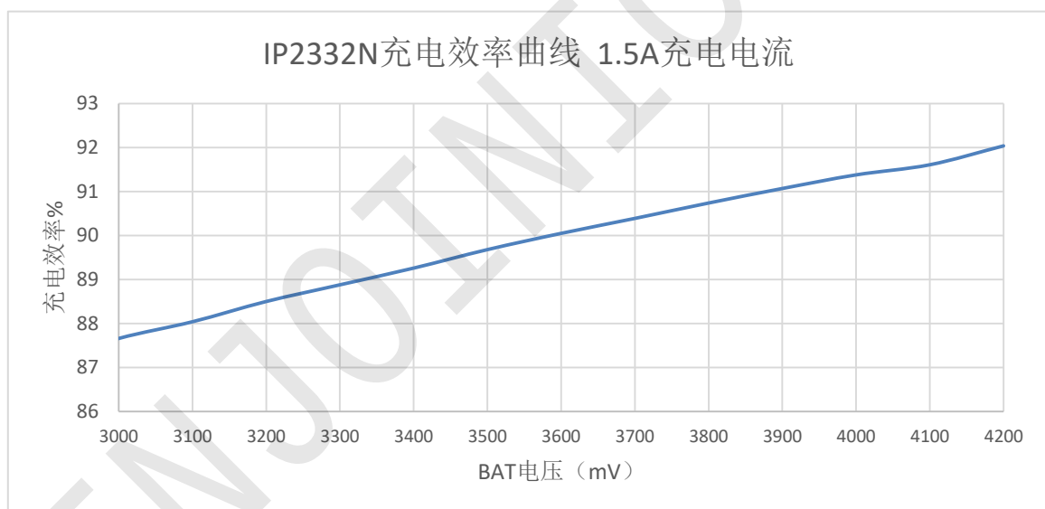
图 5 IP2332N 1.5A 充电效率曲线
