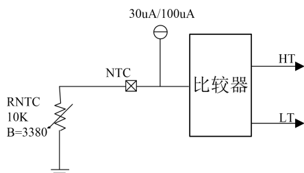
图 6 NTC 比较器
