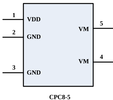
图 2：引脚图
