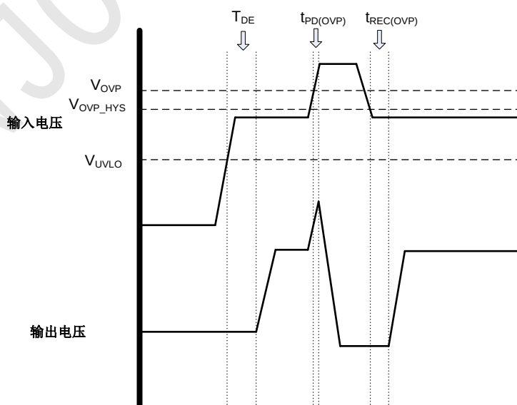
图 4 时序图
