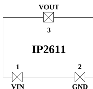
图 2 IP2611 引脚图
