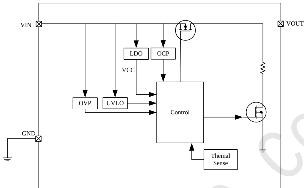
图 3 IP2617 内部系统框图
