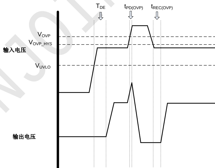
图 4 时序图
