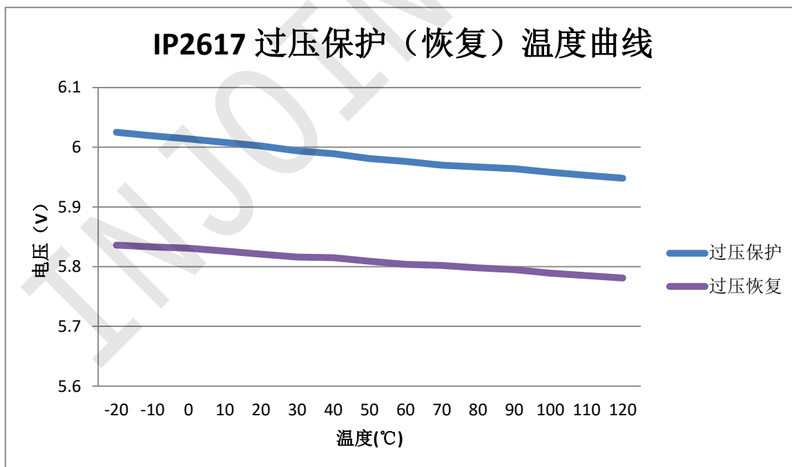
图10 过压保护（恢复）温度曲线
