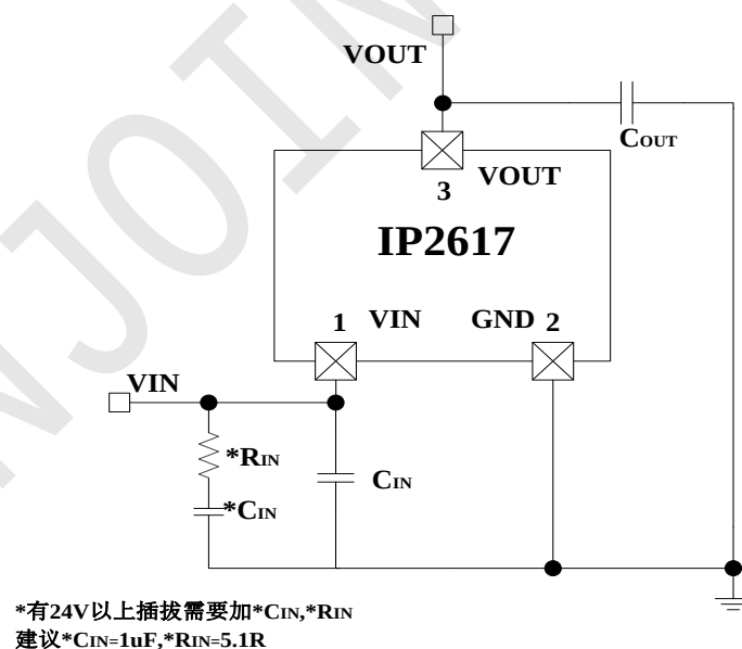
图 1 IP2617 简化应用原理图
