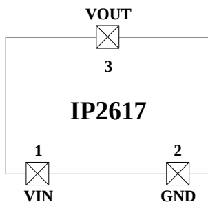
图 2 IP2617 引脚图
