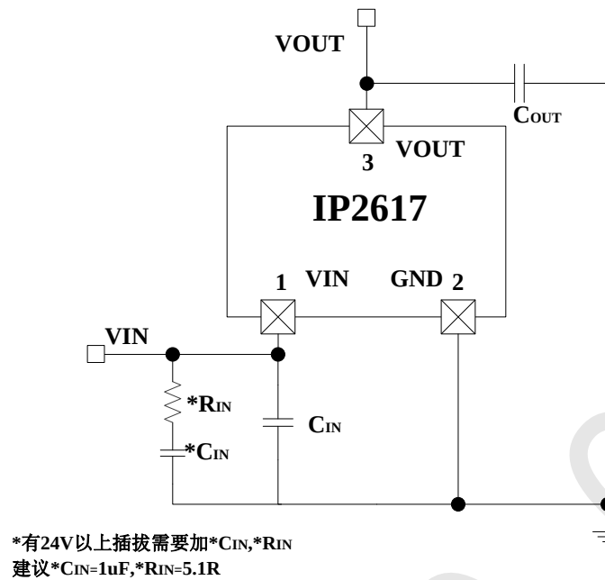
图 11 典型应用原理图
