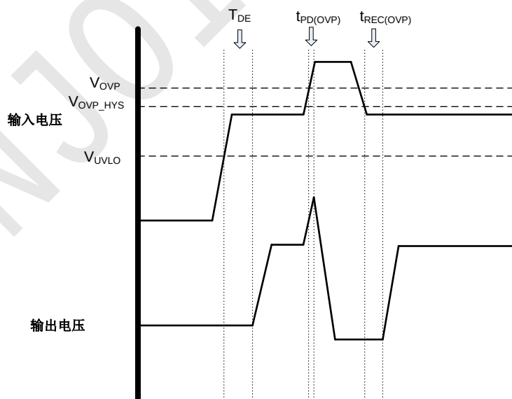
图 4 时序图
