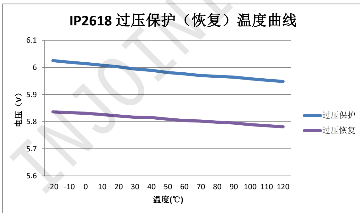
图 8 过压保护（恢复）温度曲线
