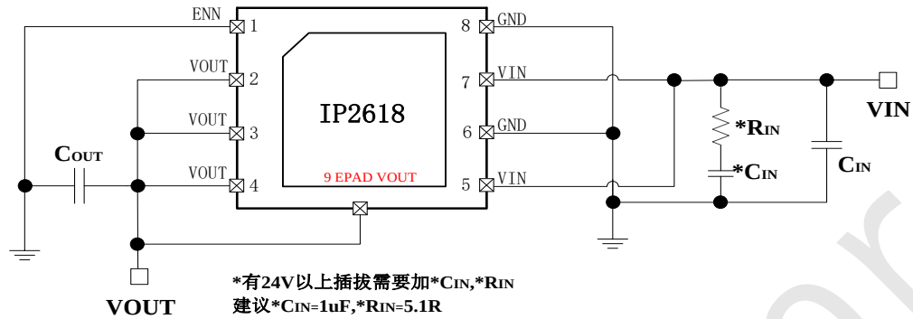
图 9 典型应用原理图
