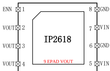
图 2 IP2618 引脚图
