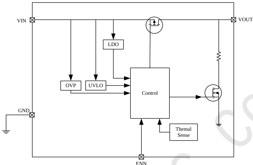
图 3 IP2618 内部系统框图
