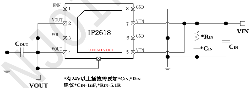
图 1 IP2618 简化应用原理图
