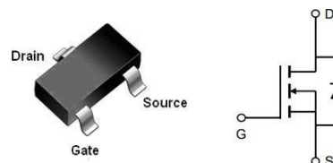
SOT23
