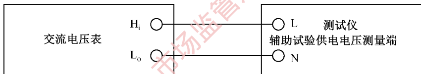
图7 带试验电压源输出的试验电压示值误差测量设备连接示意图
