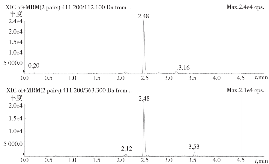
图 A.1 空白牛肝脏基质匹配标准溶液中吡利霉素特征离子质量色谱图(1.6 ng/mL)
