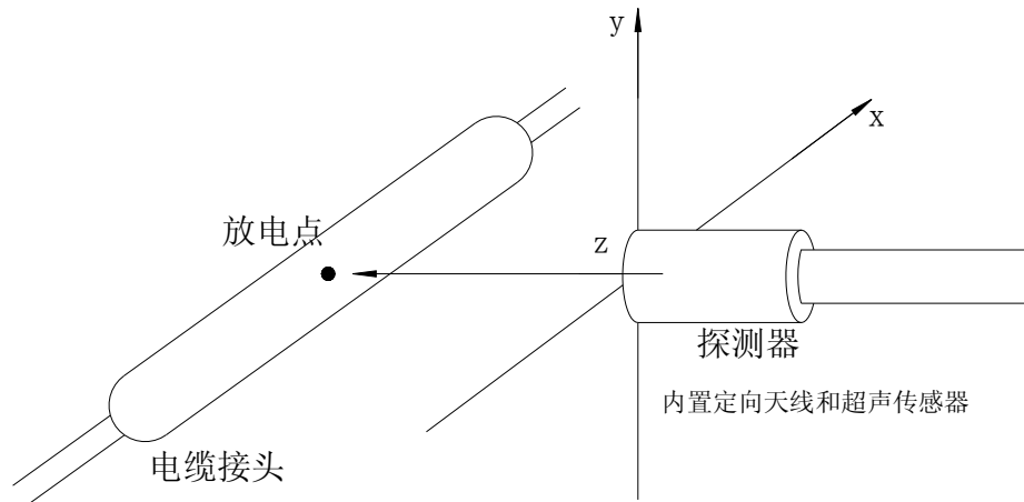
图9-2 局放定位探测器定位原理
