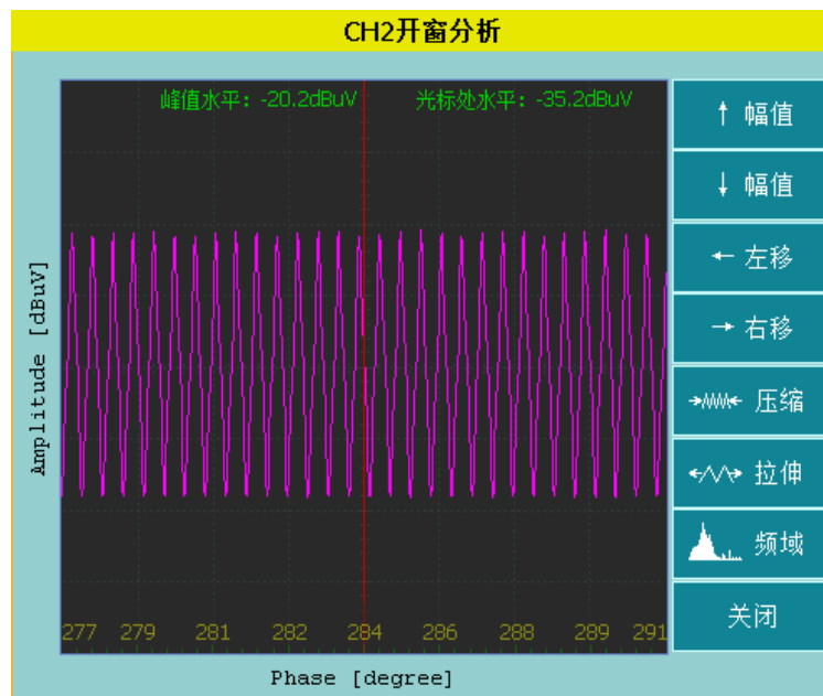
图5-17 开窗分析
