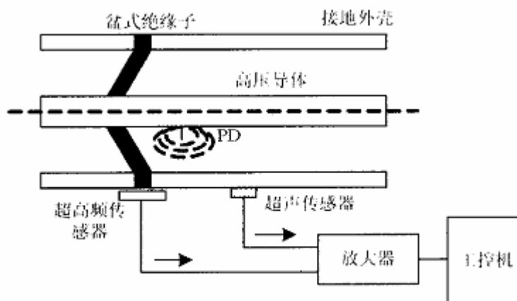
图7-3 UHF 和超声波联合检测
