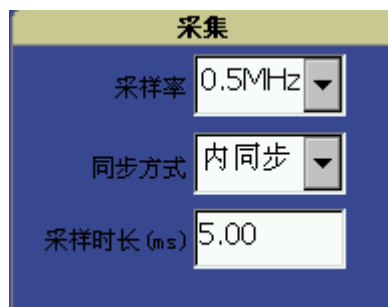
图12-3 采集设置
