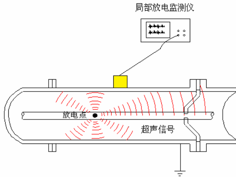
图7-2 超声波法检测原理
