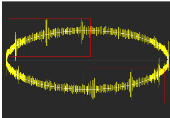
图9-5 发生较强放电
