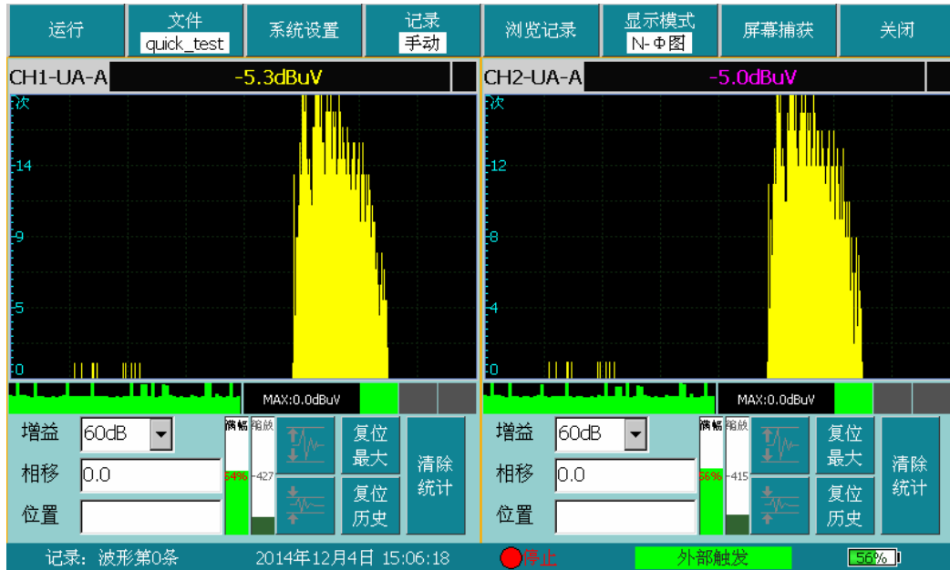
图5-12 N- \Phi 图模式
