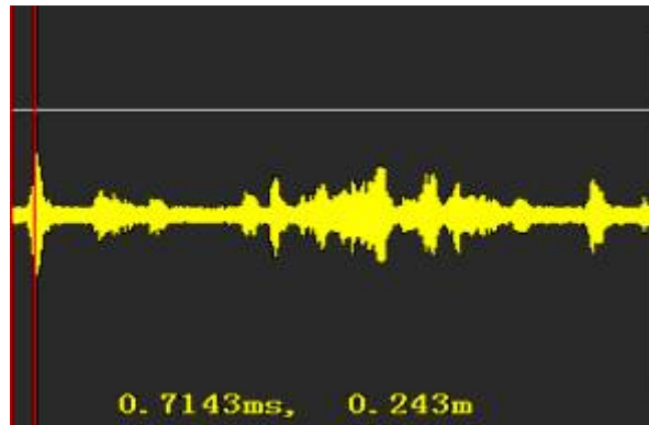
图9-7 发生严重放电（声信号）
