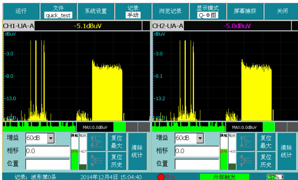
图5-13 Q- \Phi 图模式
