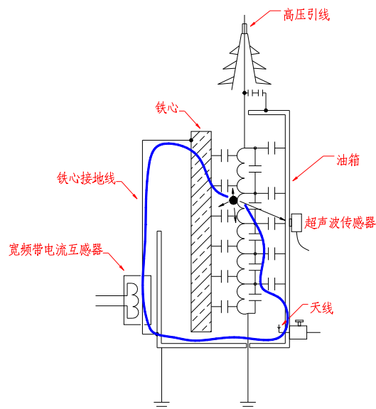
图8-2 局放信号取样示意图
