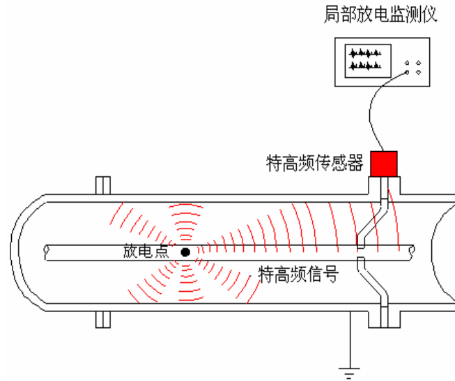
图7-1 特高频检测原理
