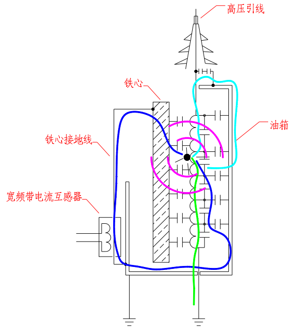
图8-1 局放信号传播途径
