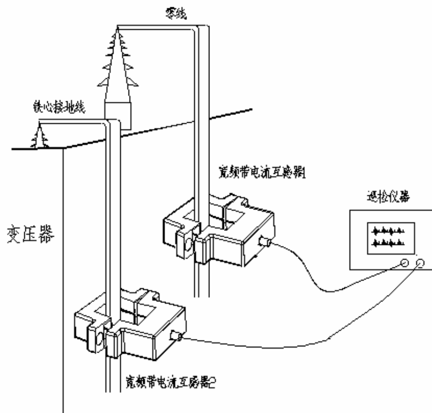
图8-3 HFCT 检测位置
