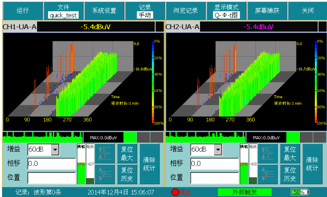
图5-14 Q-Φ-T 图模式
