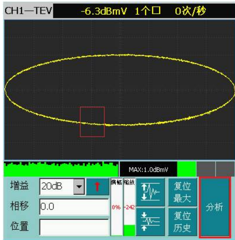
图5-16 开相位窗并进行单脉冲分析
