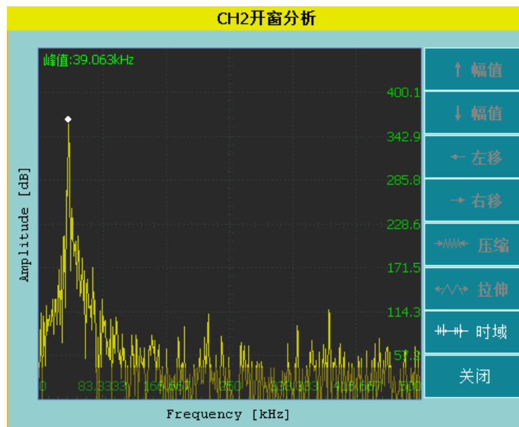
图5-18 频谱分析窗口
