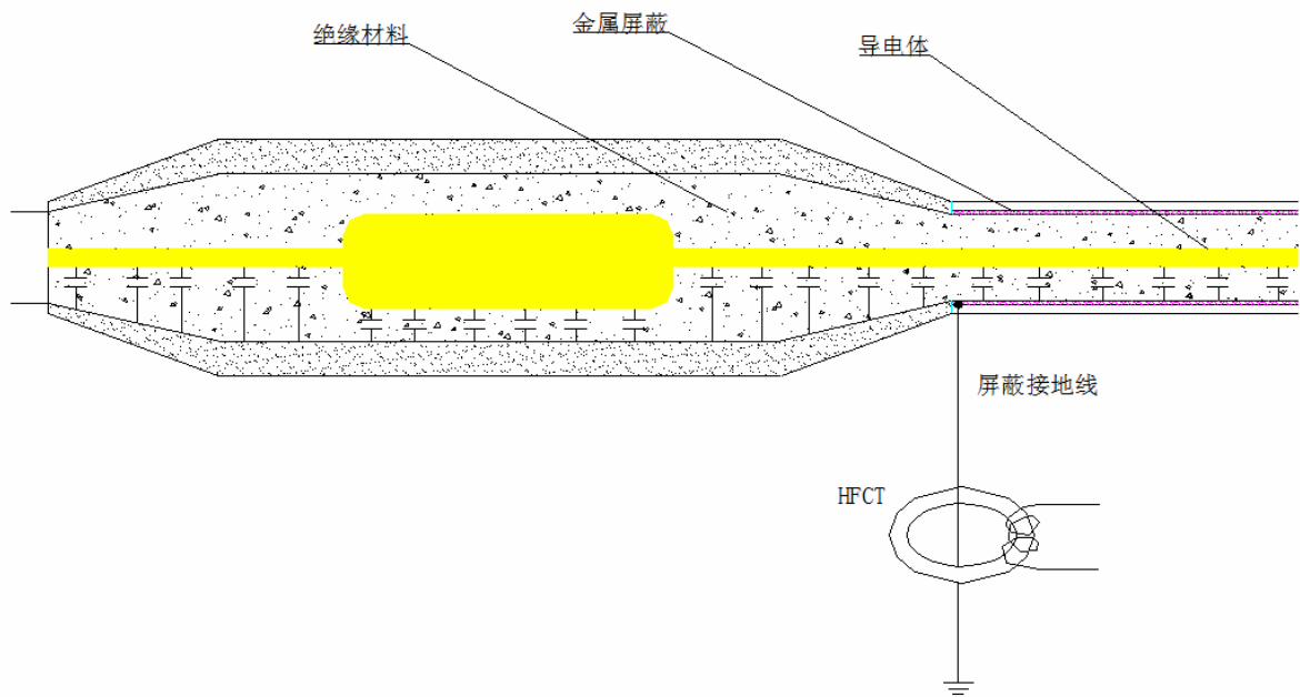
图9-1 电缆检测原理
