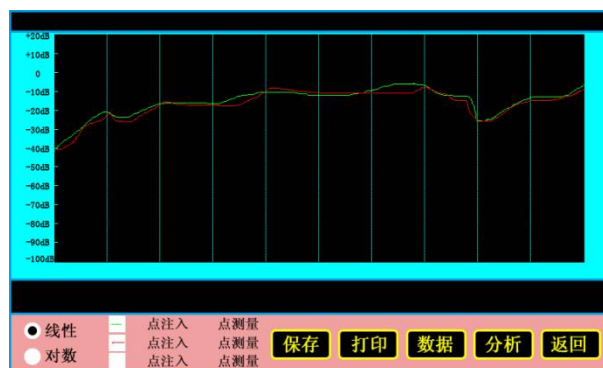
图 10 测试结果界面
