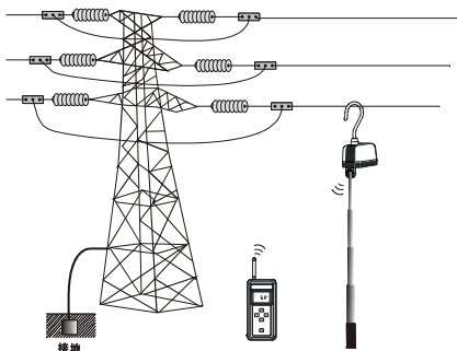
现场测试示意图
