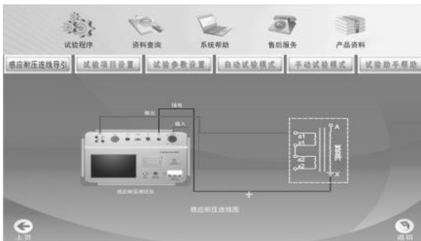
二次绕组串联加压连线图（无分压器）
