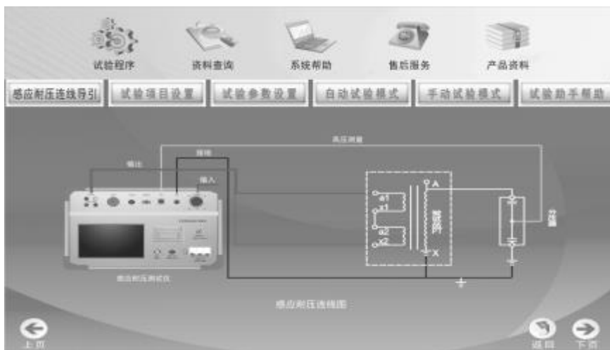
二次绕组串联加压连线图（有分压器）
