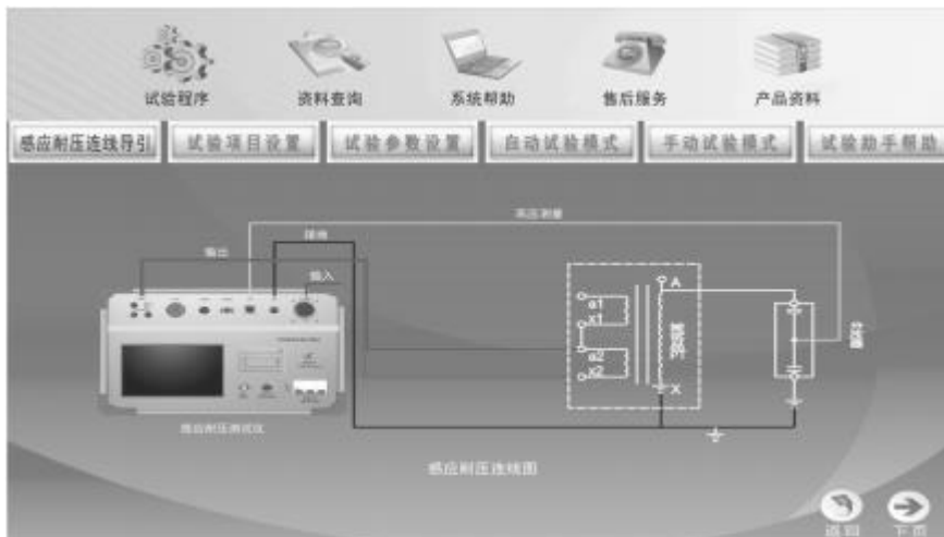
二次绕组加压连线图（有分压器）
