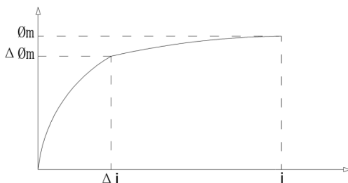
图 1 激励电流与主磁通振幅
