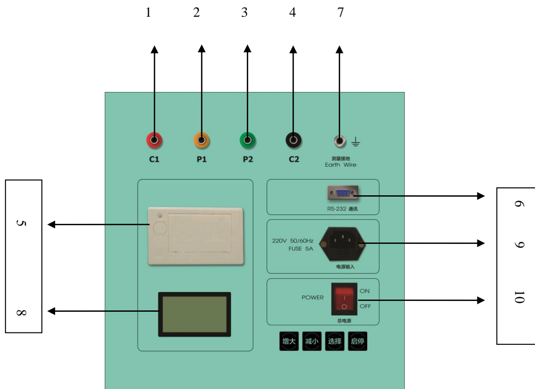
电源主机面板示意图
