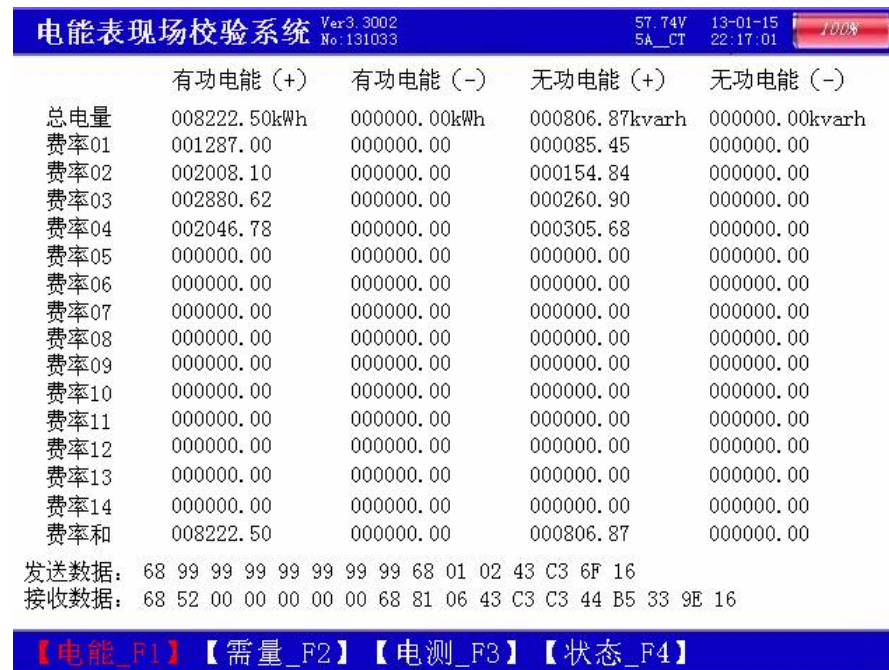
图十二、测试_485 电能
