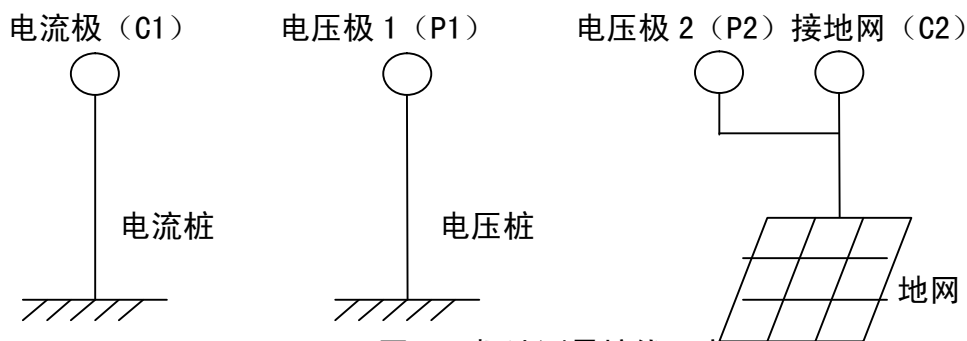
图 2 三极法测量接线示意图
