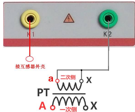
图 32，PT 交流耐压接线图
