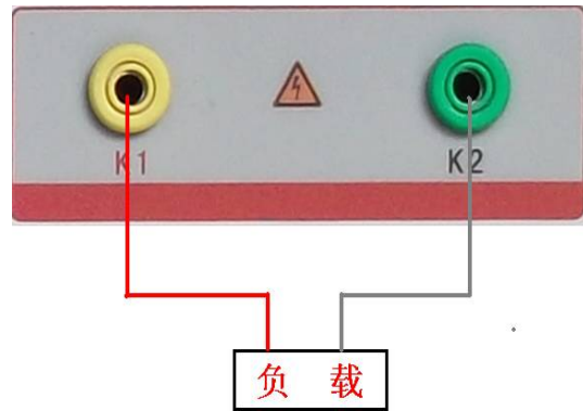
图 34，CT 二次负荷接线图
