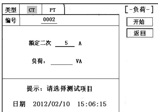
图 19, CT 二次负荷测试界面
