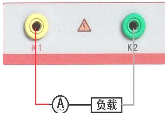
图 25, 电压校准接线图
