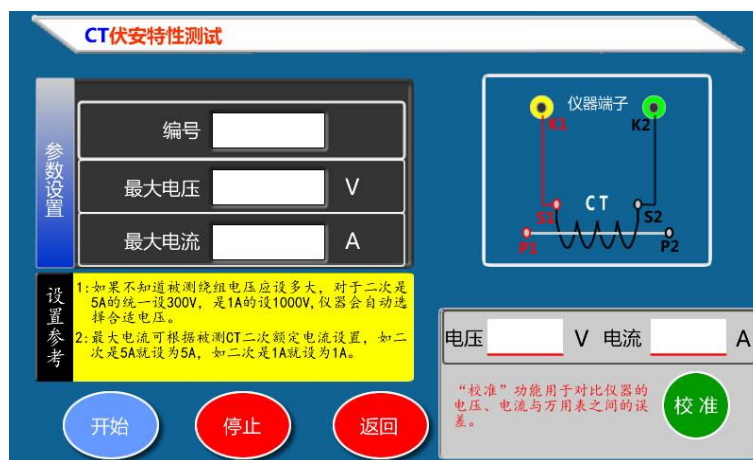
图 4，CT 励磁特性测试界面
