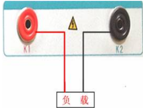
图 35，PT 二次负荷接线图
