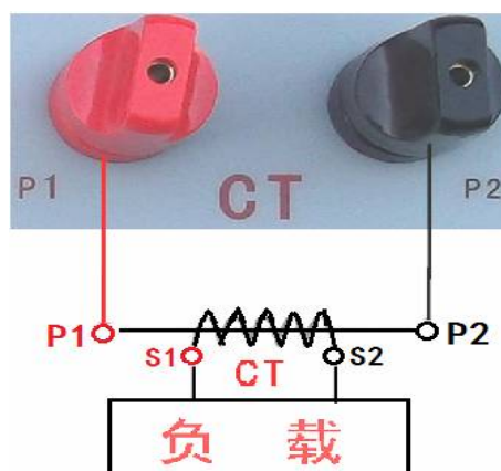
图 17、CT 一次通流接线图
