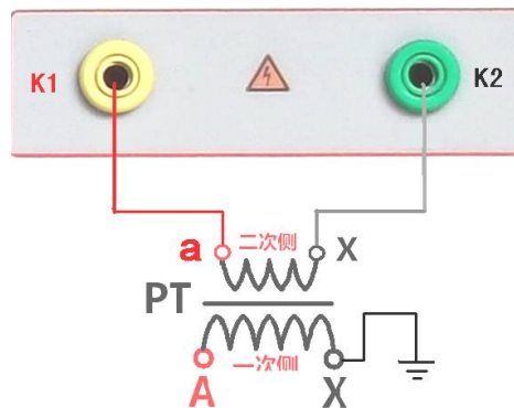
图 26，PT 励磁特性接线图
