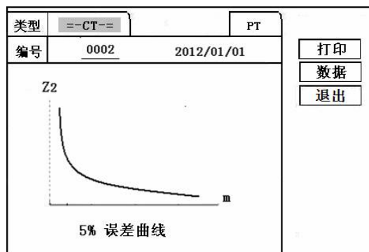
图 9, 误差曲线图
