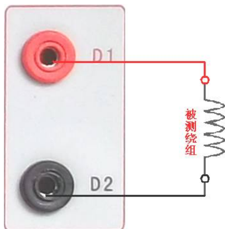
图 24，直阻测试接线图
