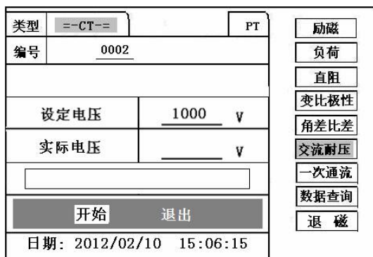
图 18, CT 交流耐压测试界面
