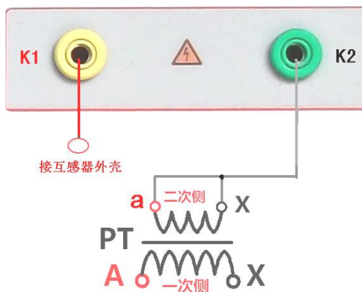
图 33， PT 交流耐压接线图
