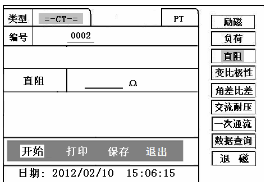
图 22，直阻测试界面
