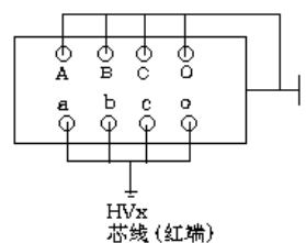
图14 变压器接法
