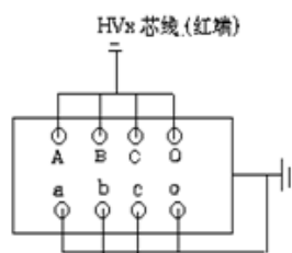
图13 变压器接法
