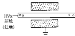
图11 套管接法
