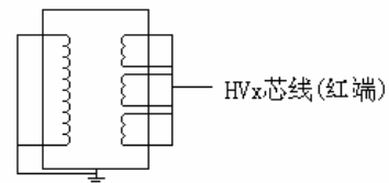
图8 PT接法
