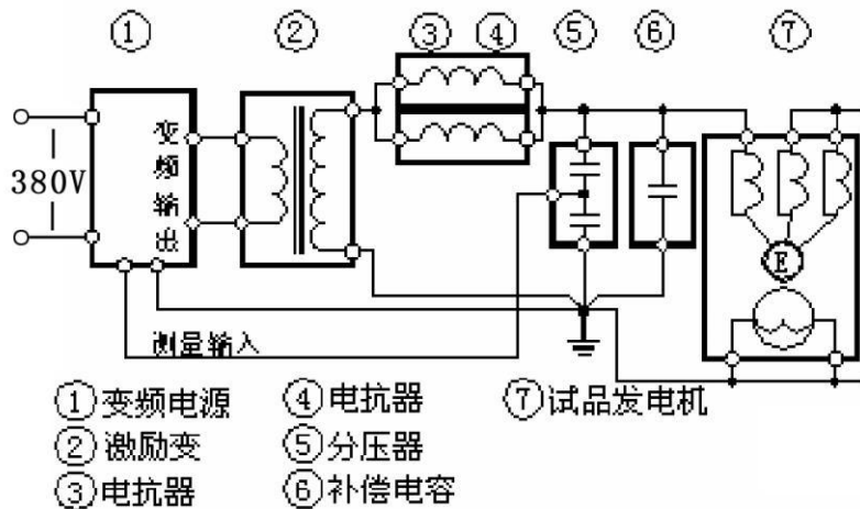
发电机耐压试验接线图
