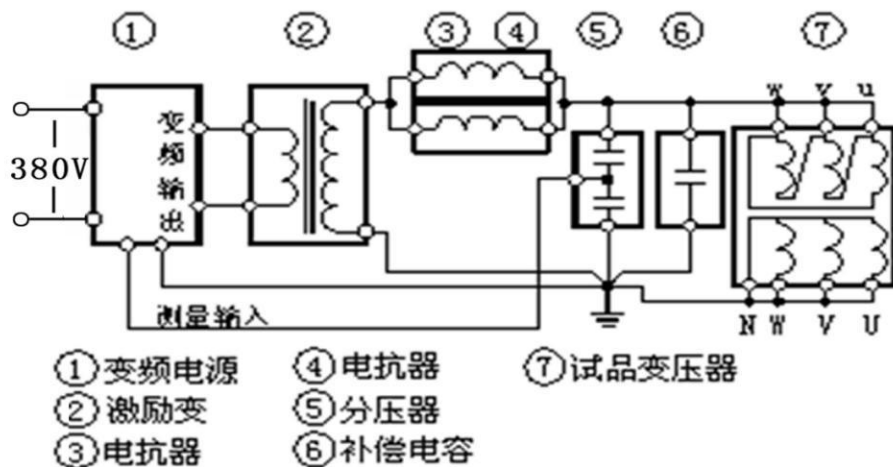
变压器耐压试验接线图
