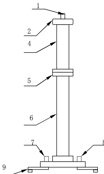
图 5 双节倍压筒
