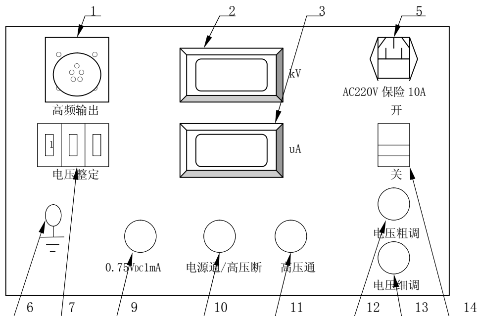
图3 LYZGS 直流高压发生器控制箱面板示意图(单节倍压)
