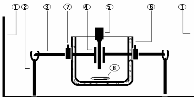
图二 高压舱内布置图
